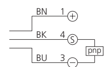
Empfänger / receiver
