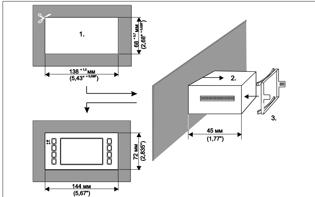
Рис. 20: Панельный монтаж
