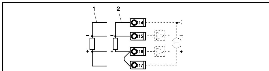
Рис. 19: Подключение датчика температуры, дополнительная карта расширения для температуры, например, в гнезде В (гнездо В I)
