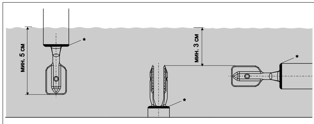
Рис. 9: Зубцы вилки и "*" мембрана должны быть полностью покрыты продуктом.
