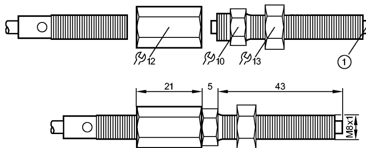
1: подвижный штифт с возвратной пружиной (ход: 1,5 мм, Ø 5,5mm)
