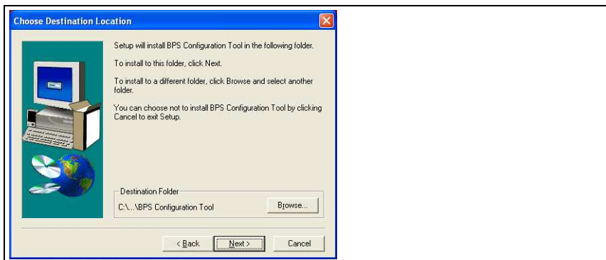
Рис. 8.5: Установочная папка
