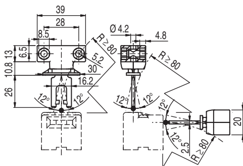
Рис. 13.6: Контактный элемент АС-АН-F4J2-ТК
