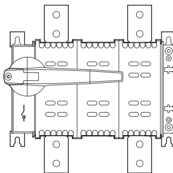
DDC-1000/2-SK DDC-1250/2-SK
