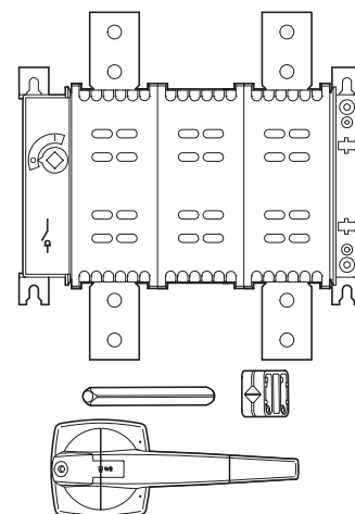
DDC-1000/2/M4/P-G DDC-1250/2/M4/P-G
