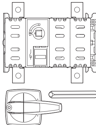
DDC-125/2/M4/P-G, DDC-160/2/M4/P-G, DDC-200/2/M4/P-G
