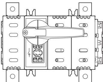
DDC-250/2, DDC-400/2, DDC-630/2
