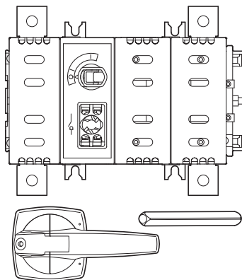
DDC-250/2/M4/P-G, DDC-400/2/M4/P-G, DDC-630/2/M4/P-G
