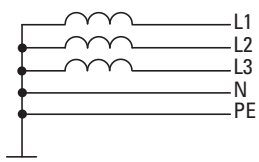
TN-S
