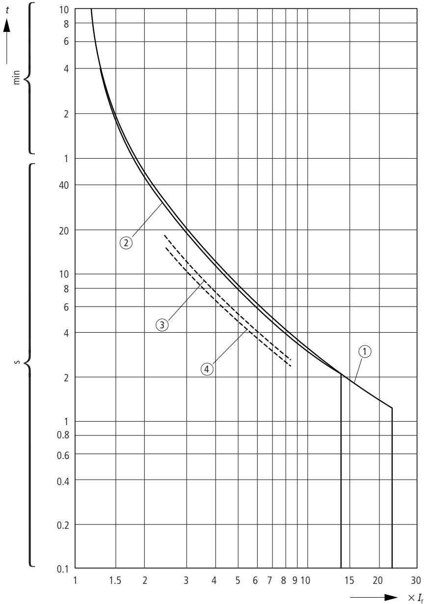
Abbildung/Figure 10: PKZM0-0,16/XTPRP16BC1
