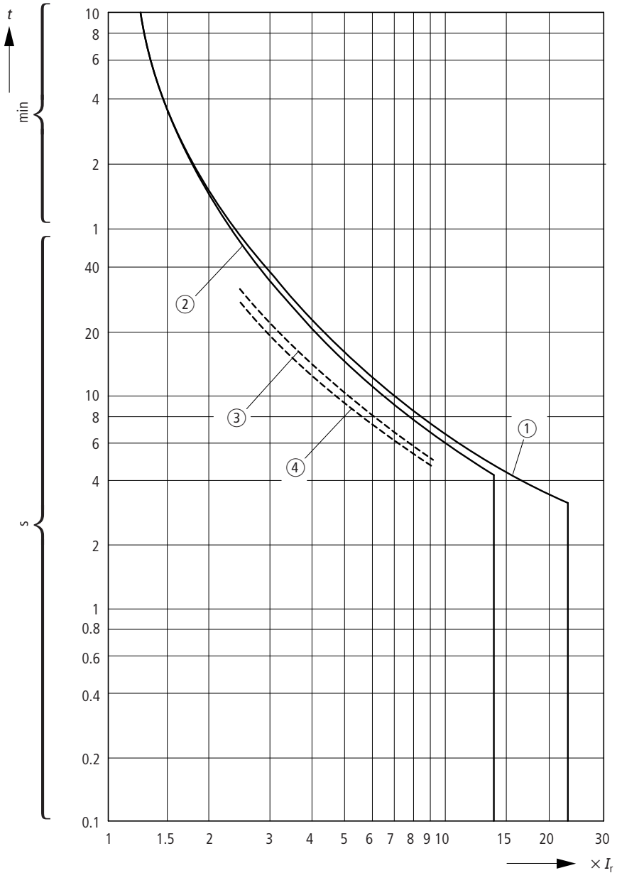
Abbildung/Figure 16: PKZM0-2,5/XTPR2P5BC1
