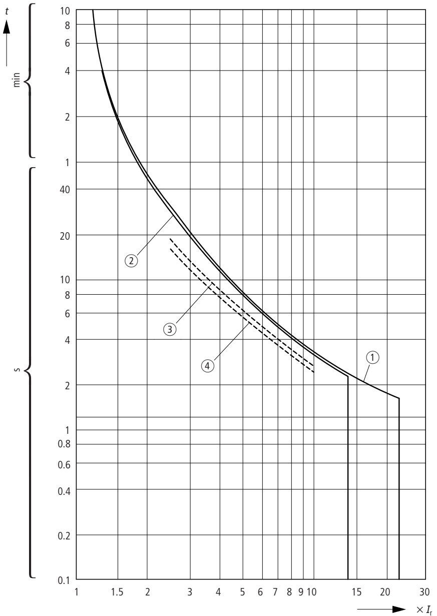
Abbildung/Figure 11: PKZM0-0,25/XTPRP25BC1
