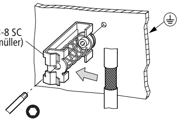
Figura 10: Schermatura della linea di rete
