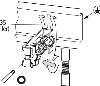
Figura 10: Schermatura della linea di rete
