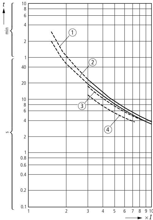
Abbildung/Figure 15: ZE-0,4/XTOMP40AC1
