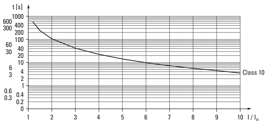
Abbildung 8: Auslösekennlinie für Nennstromeinstellung bis 4 A
