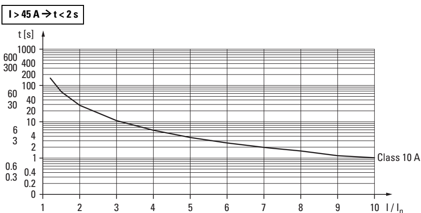
Abbildung 9: Auslösekennlinie für Nennstromeinstellung größer als 4 A
