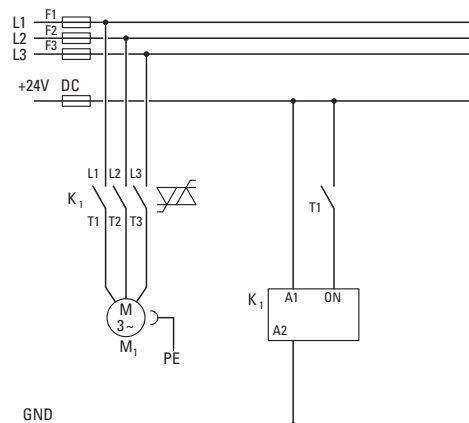
Abbildung 2: Direktstarter
