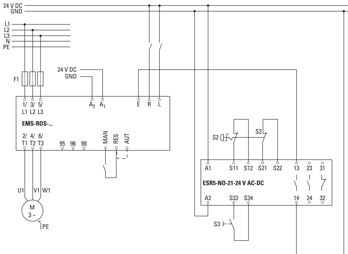
Abbildung 6: Haupt- und Steuerstrompfad NOT-HALT (einkanalig) S2 = NOT-HALT, S3 = Reset
