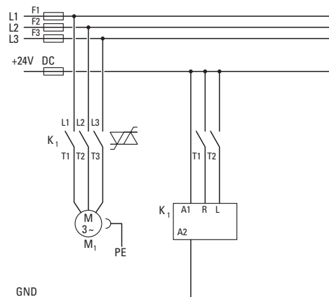
Abbildung 3: Wendestarter
