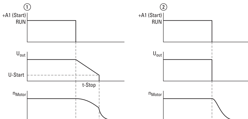
Abbildung 72: Betrieb mit ① und ohne ② Softstopp
