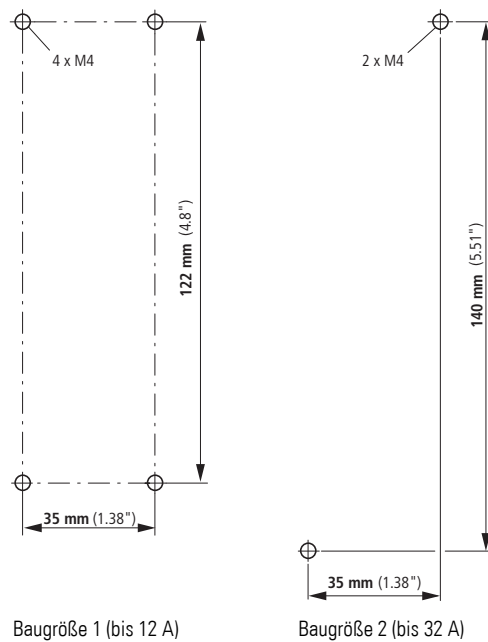
Abbildung 52: Bohrmaße
