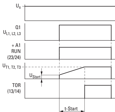
Abbildung 100: Ablaufdiagramm – ohne Softstopp
