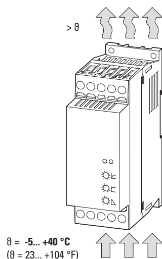
Abbildung 39: Kühlluftzufuhr
