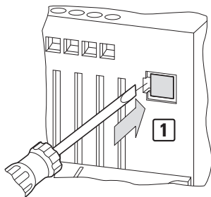
Abbildung 46: Schlitzschraubendreher in die Öffnung einführen
