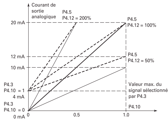
Figure 53. Mise à l'échelle de la sortie analogique
