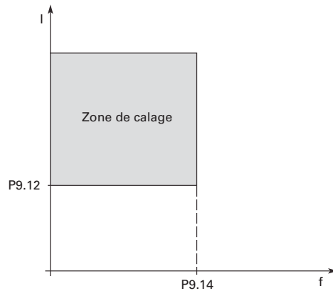
Figure 64. Réglage des caractéristiques de calage
