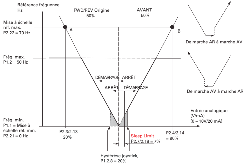
Figure 46. Exemple de la fonction de limite reste
