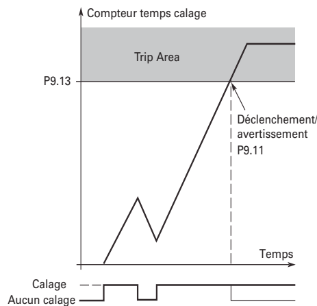
Figure 65. Comptage du temps de calage
