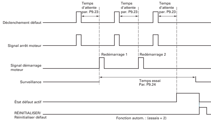
Figure 68. Exemple de redémarrages automatiques avec deux redémarrages
