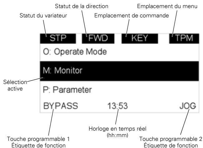
Figure 5. Vue générale de l'afficheur à cristaux liquides
