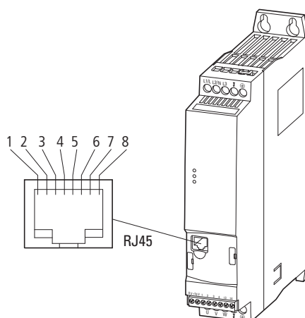
Abbildung 56: RJ45-Schnittstelle
