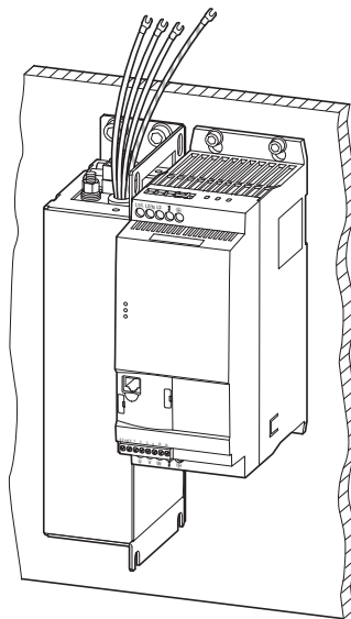
Abbildung 89: Montageanordnung (Beispiel: DX-EMC34-019... und DE1...-340... in Baugröße FS2)
