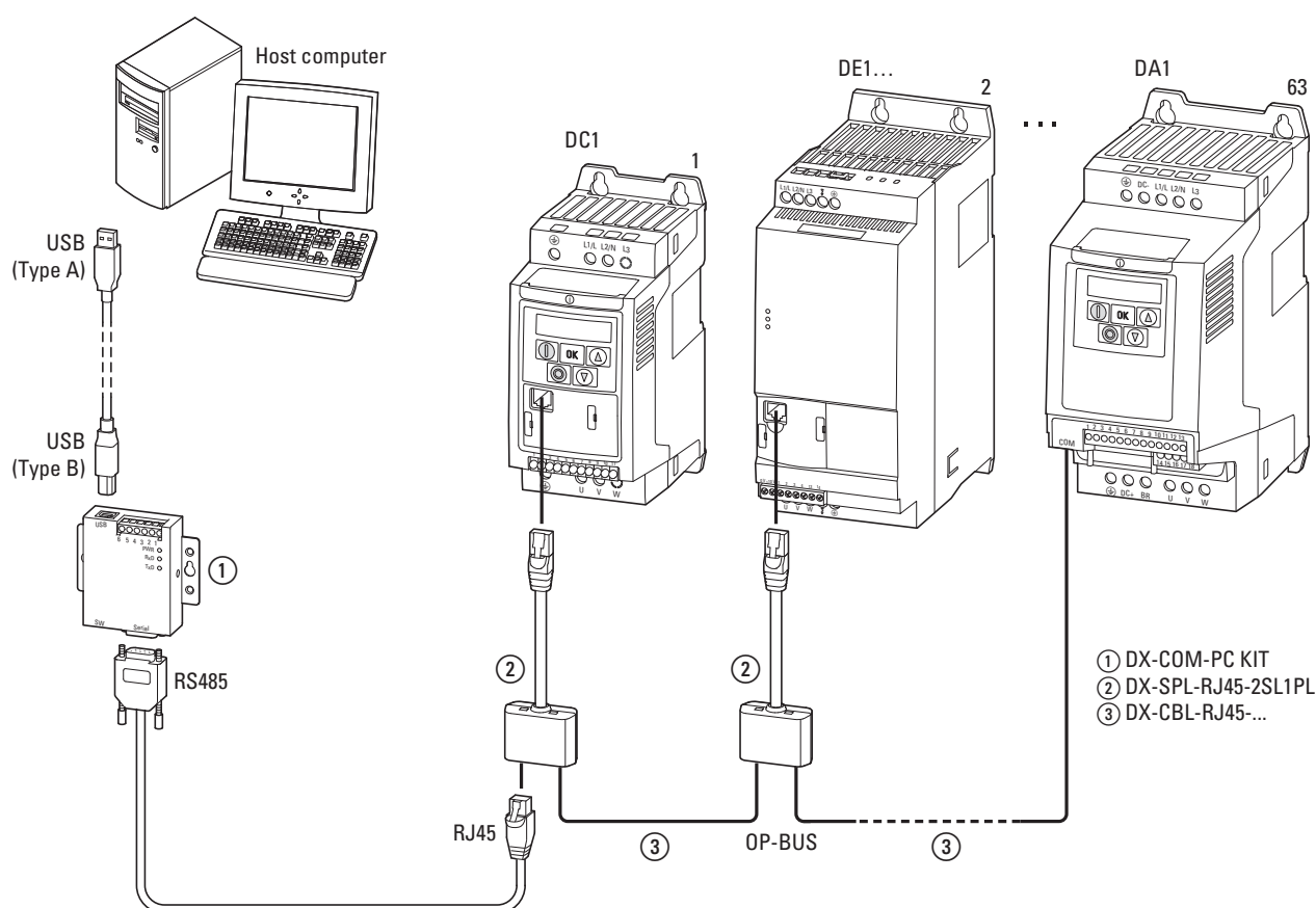
Abbildung 83: Beispiel Kommunikationsstrang
