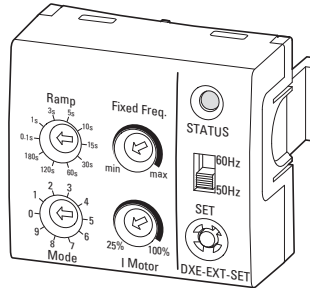
Abbildung 52: Konfigurationsmodul DXE-EXT-SET
