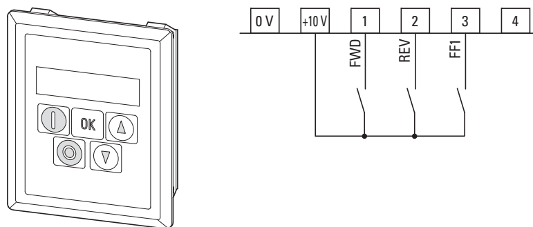
Abbildung 70: Optionale Bedieneinheit DXE-KEY-LED und Steuerklemme P-15 = 0 (Werkseinstellung, Mode 0)
