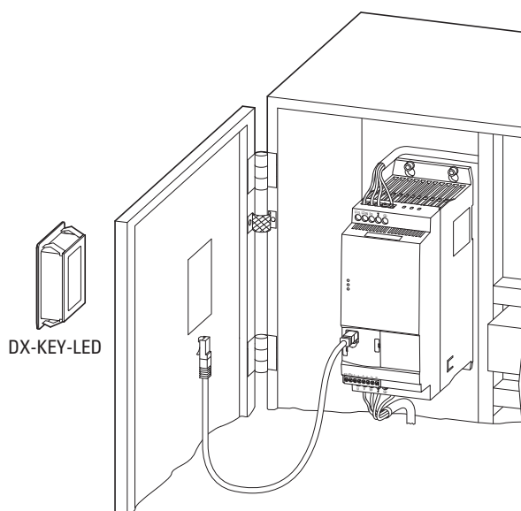
Abbildung 75: Montage in einer Schaltschranktür
