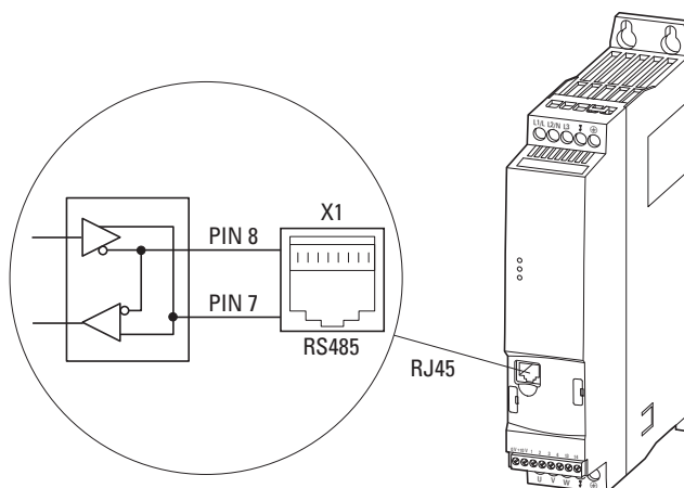
Abbildung 45: RJ45-Schnittstelle
