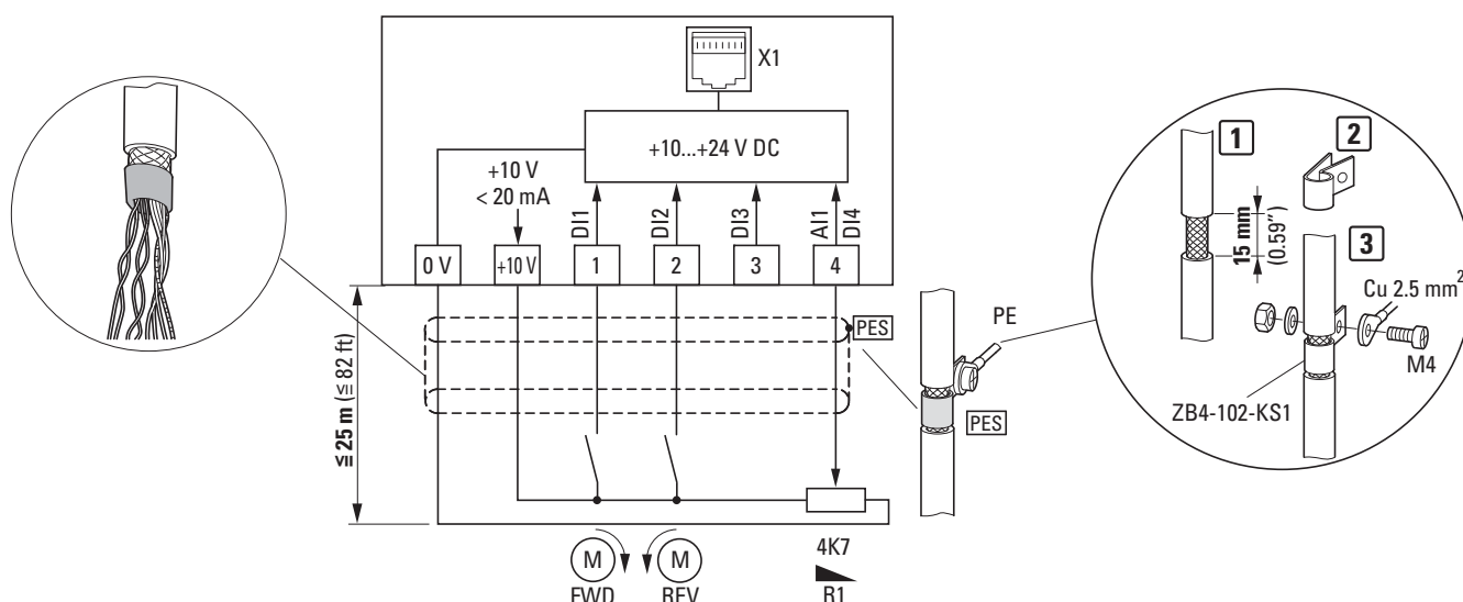
Abbildung 41: Anschlussbeispiel Steuerklemmen
