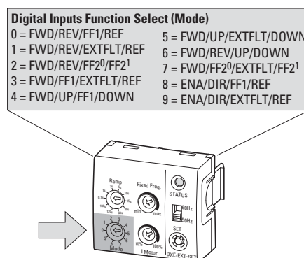
Abbildung 69: Konfigurationsmodul DXE-EXT-SET
