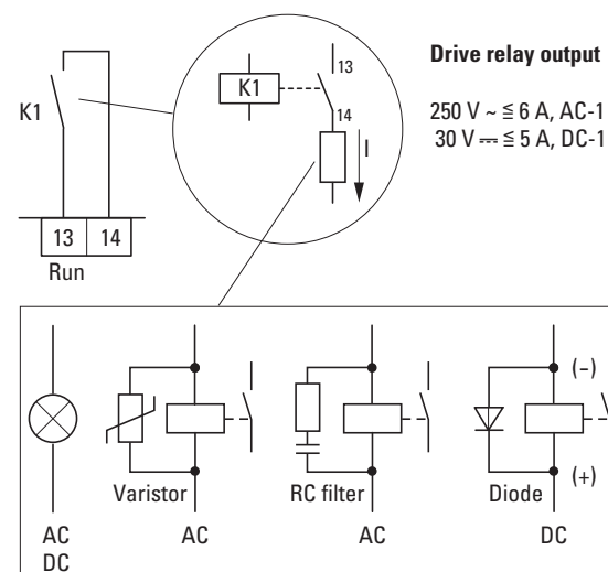
Abbildung 44: Anschlussbeispiele mit Schutzbeschaltung
