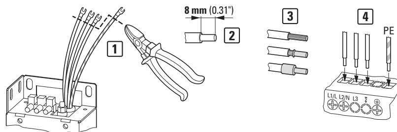
Abbildung 90: Anpassung der konfektionierten Anschlussleitungen
