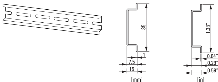
Abbildung 26: Montageschiene gemäß IEC/EN 60715
