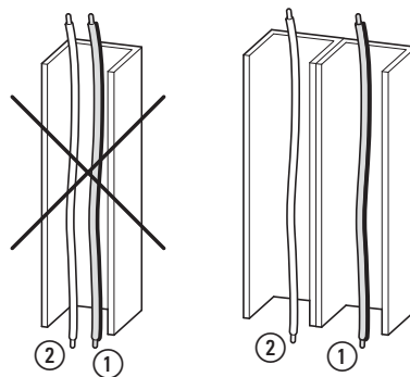
Abbildung 18: Getrennte Leitungsverlegung
