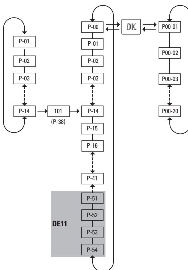
Abbildung 59: Parameterstruktur
