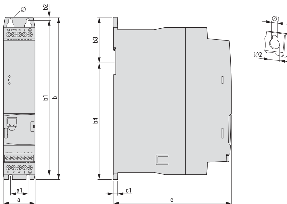
Abbildung 73: Abmessungen
