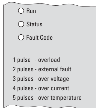
Abbildung 92: LED-Anzeigen mit Fehlermeldung
