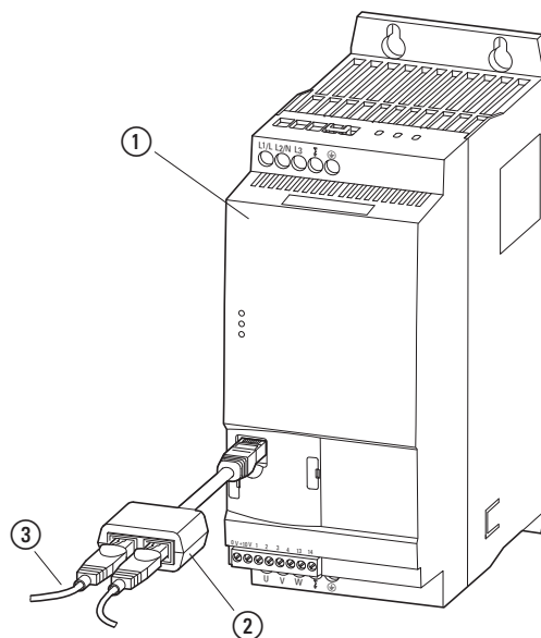
Abbildung 85: RJ45-Anschluss
