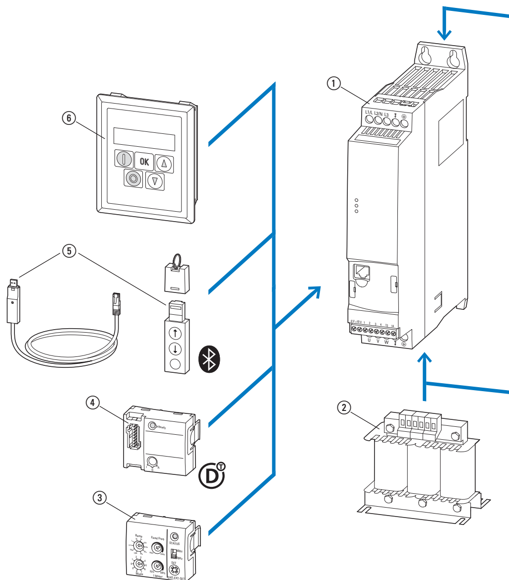
Abbildung 2: Systemübersicht (Beispiel)
