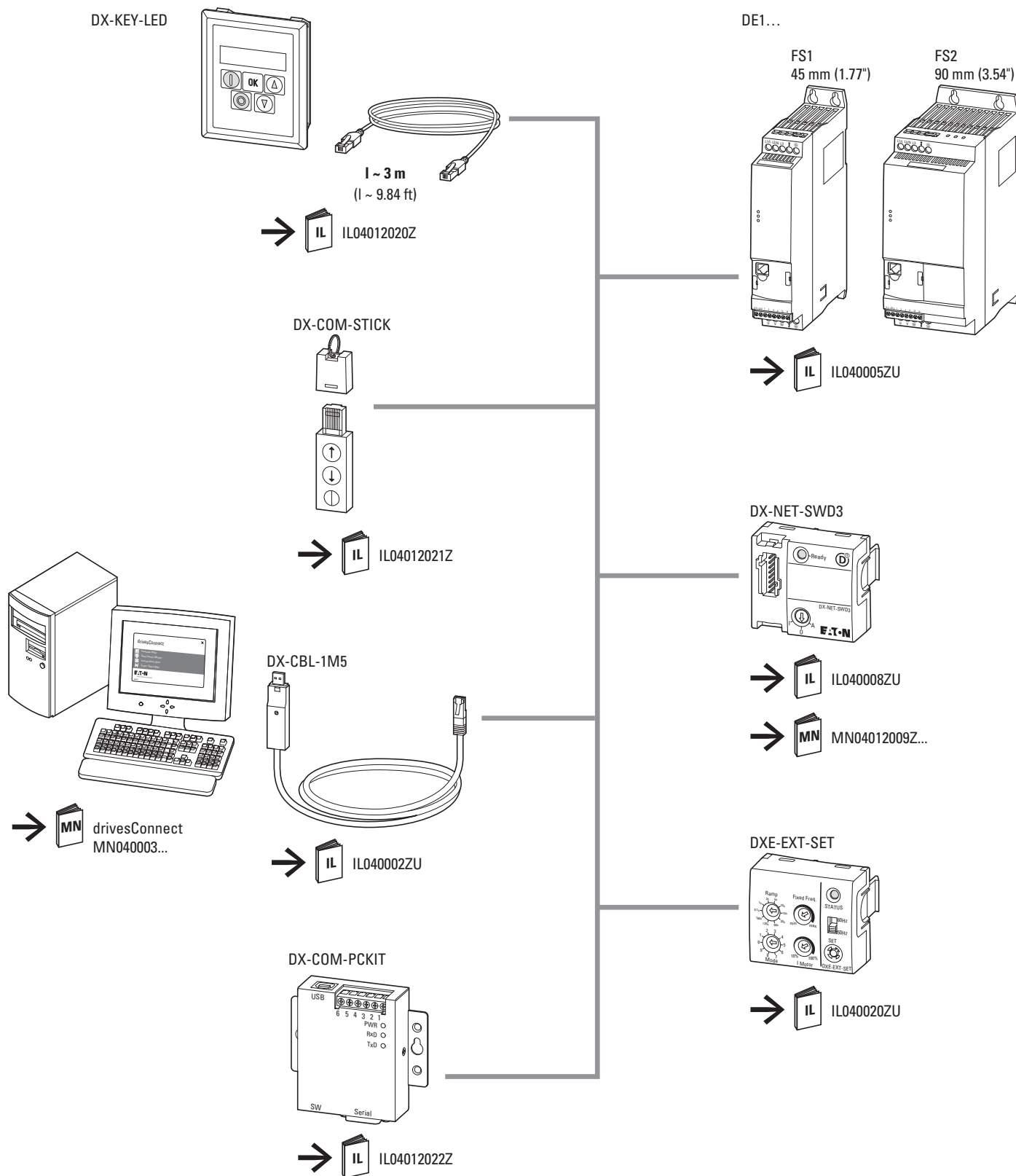
Abbildung 46: Systemübersicht zur RJ45-Schnittstelle des Drehzahlstarters DE1
