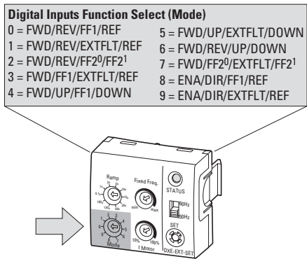
Figura 69: Modulo di configurazione DXE-EXT-SET
