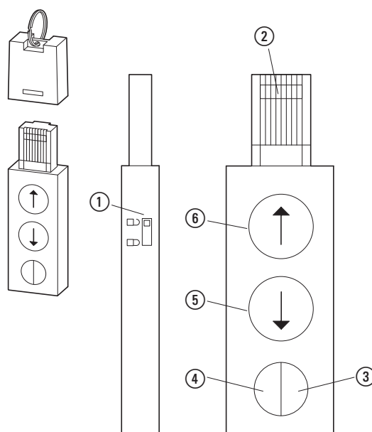
Figura 78: DX-COM-STICK
