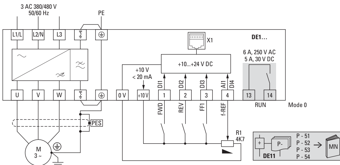
Figura 50: Schema a blocchi DE1-34...FN-...
