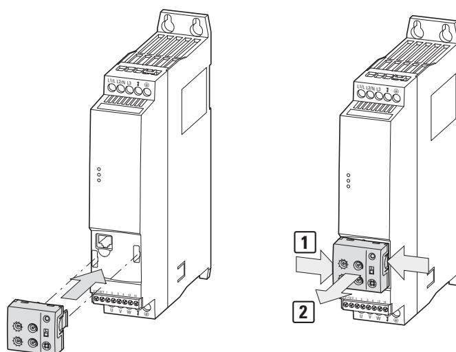
Figura 54: Montaggio e smontaggio
