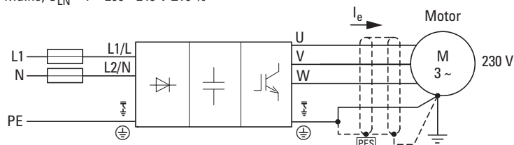
Figura 10: DE1...-12...NN-N20N (senza filtro soppressione radiodisturbi)
