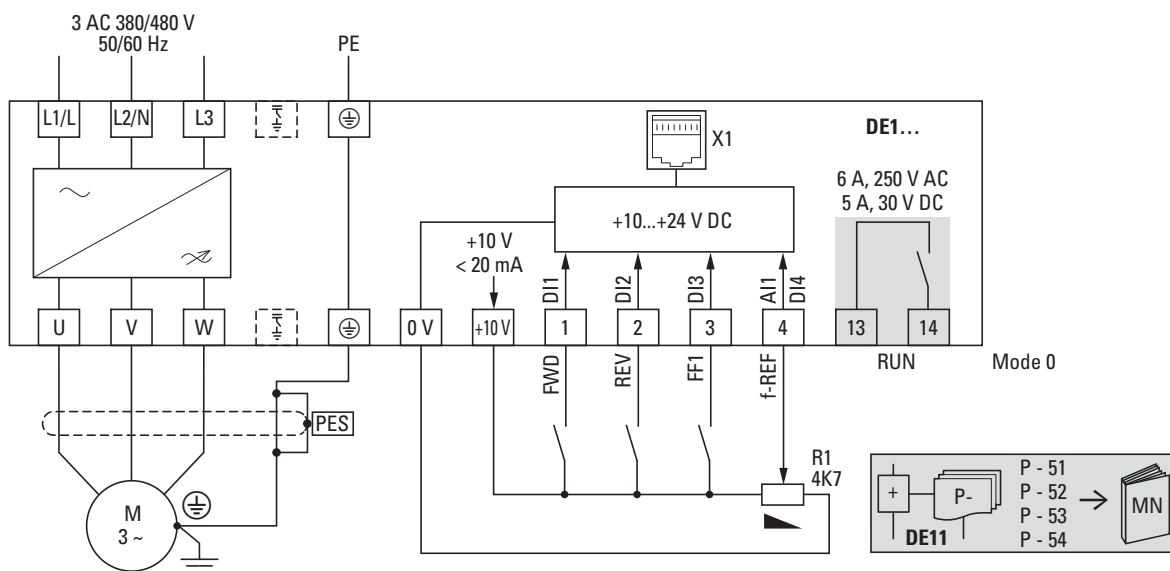
Figura 51: Schema a blocchi DE1-34...NN-...
