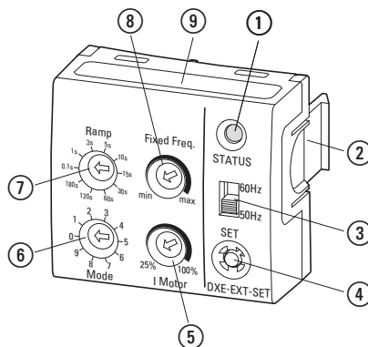
Figura 53: Designazioni su DXE-EXT-SET
