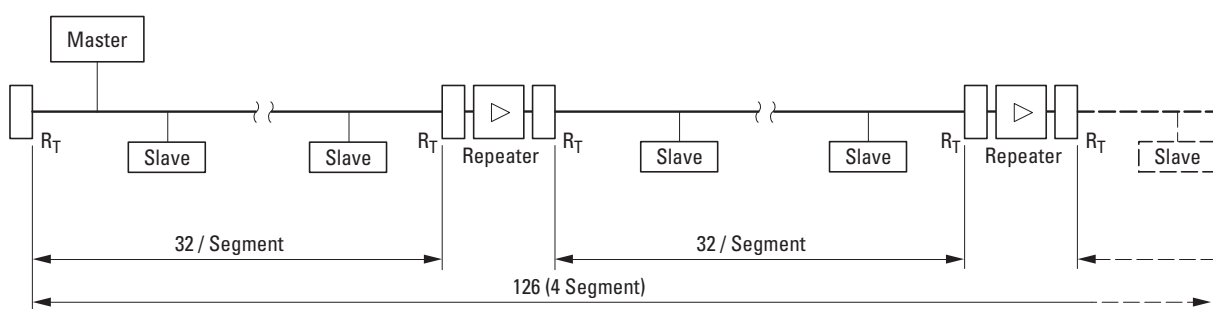
Figure 5 : Chaîne PROFIBUS DP avec 126 participants maximum répartis sur quatre segments (32 participants maximum par segment)
