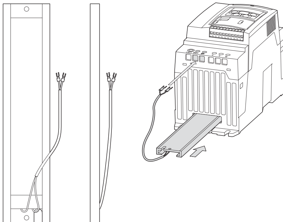
Obrázek 118: Brzdný odpor DX-BR3-100
