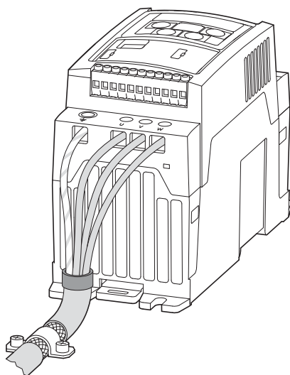
Obrázek 36: Příklad připojení
