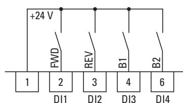
Obrázek 76: Příklad: pevné frekvence FF1 až FF4
