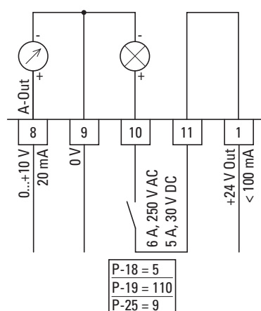
Obrázek 82: Příklad: Sledování proudu motoru Chybová zpráva: I.L - LrP
