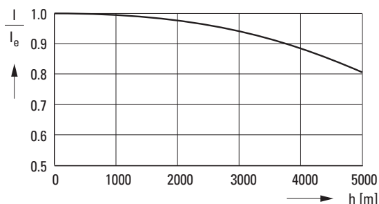
Obrázek 121: Hodnoty snížení výkonu při odlišných výškách instalace a okolních teplotách
