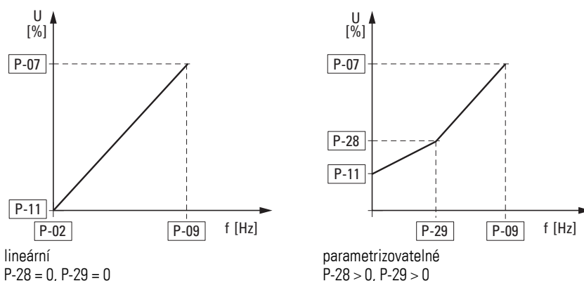
Obrázek 66: Charakteristika U/f
