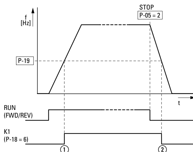
Obrázek 71: Externí brzda ovládaná přes K1
