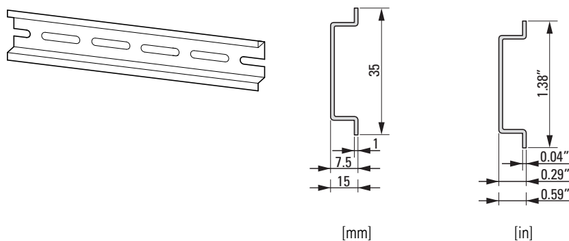
Obrázek 23: Montážní lišta podle normy ČSN EN 60715
