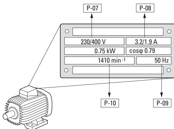
Obrázek 64: Parametry motoru z výkonového štítku
