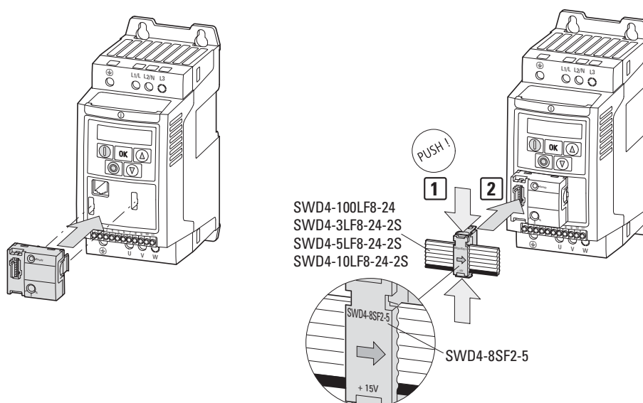
Obrázek 105: Připojení SmartWire-DT
