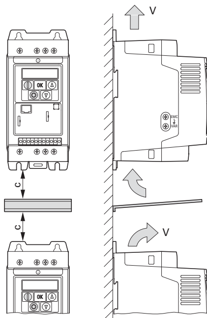
Obrázek 19: Deflektor
