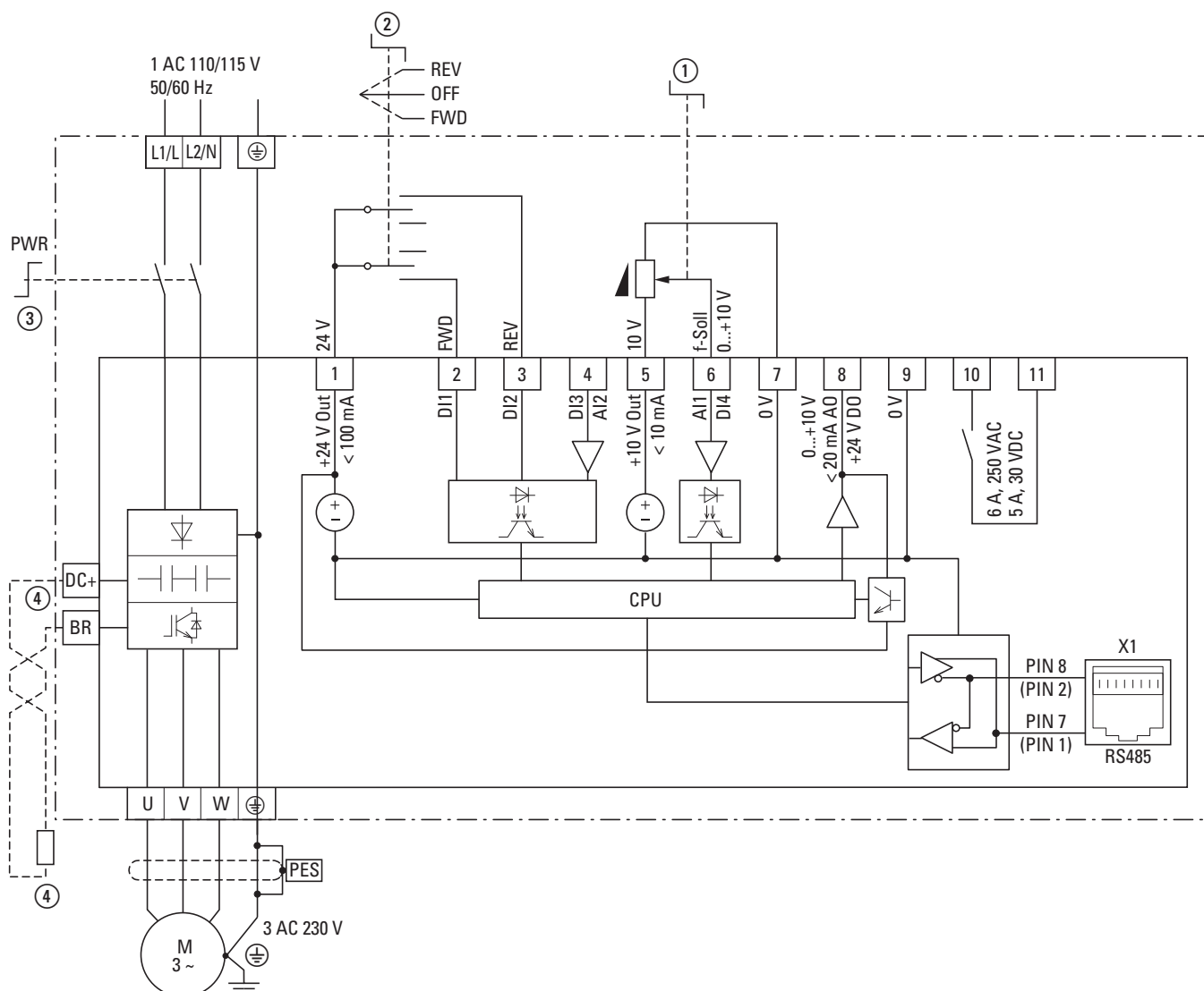
Obrázek 52: Blokové schéma DC1-1D...Nx-A6SN
