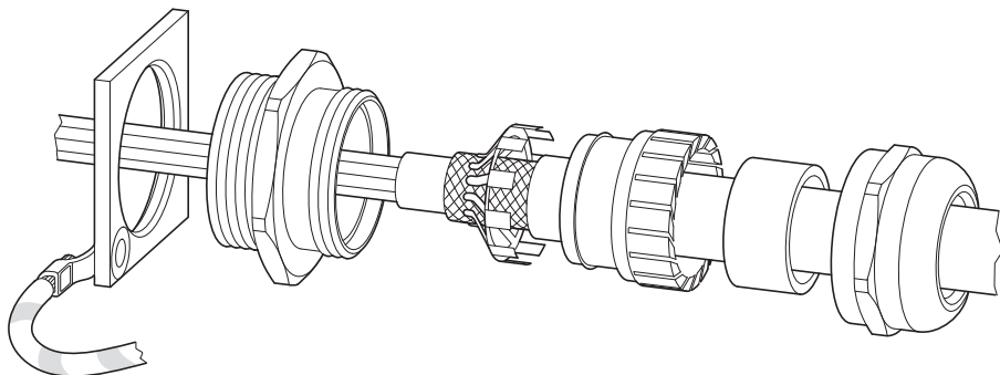
Obrázek 30: Principiální struktura kabelové průchodky EMC
