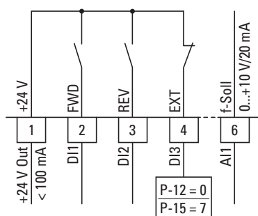
Obrázek 74: Příklad připojení: externí chyba (EXT)
