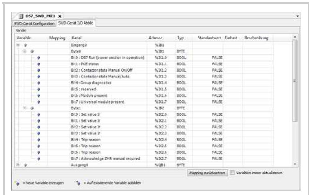
Abb. 20 Konfigurationseditor-Dialog SWD-Teilnehmer, Registerkarte [SWD-Gerät I/O Abbild]
