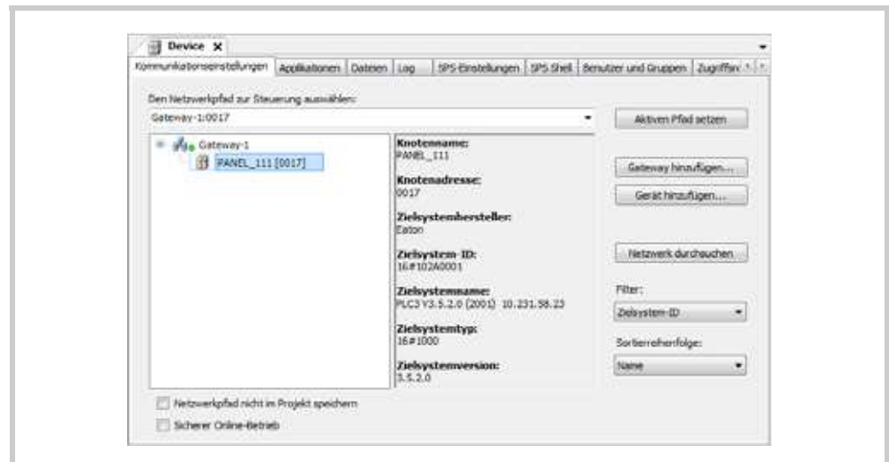
Abb. 28 Geräte-Editor, Registerkarte [Kommunikationseinstellungen]
