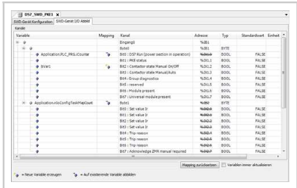
Abb. 16 Konfigurationseditor-Dialog, Registerkarte [... I/O Abbild]
