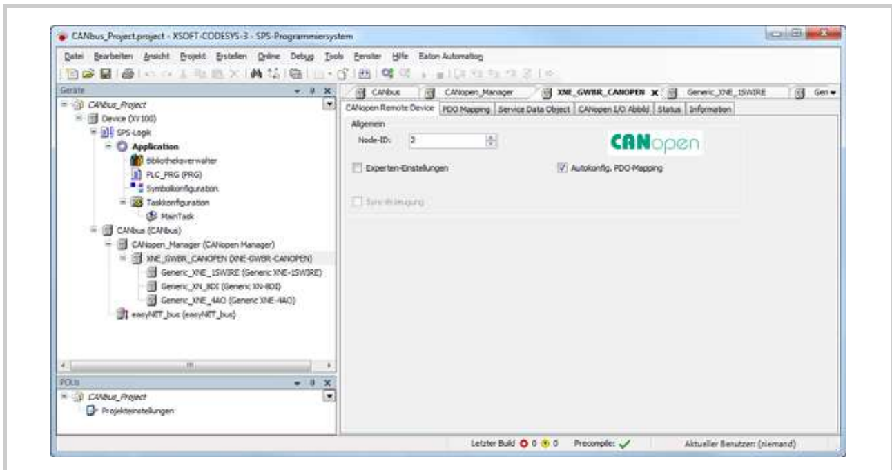
Abb. 15 Dialoge des Feldbus-Konfigurationseditors
