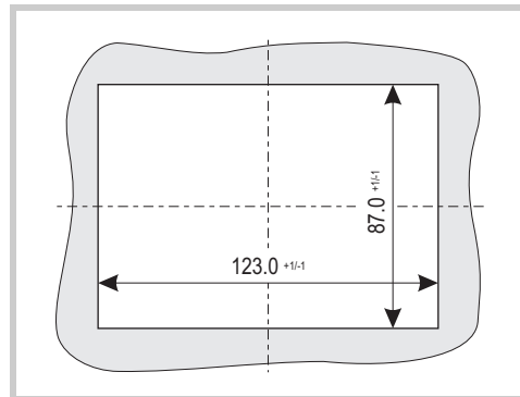
Abb. 26 Einbauausschnitt für 3,5"-Geräte
