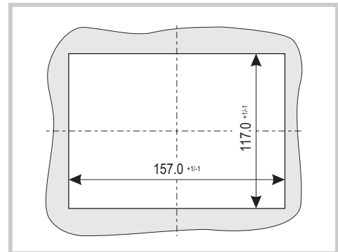
Abb. 27 Einbauausschnitt für 5,7"-Geräte
