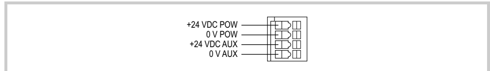
Abb. 18 Steckverbinder WAGO (Ansicht von der Verdrahtungsseite)
