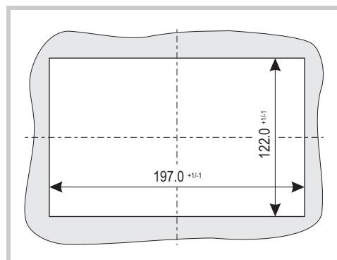
Abb. 28 Einbauausschnitt für 7,0"-Geräte
