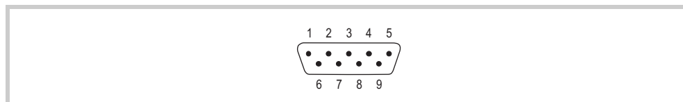
Abb. 12 RS232-Schnittstelle (9-polig, D-Sub, male, UNC)
