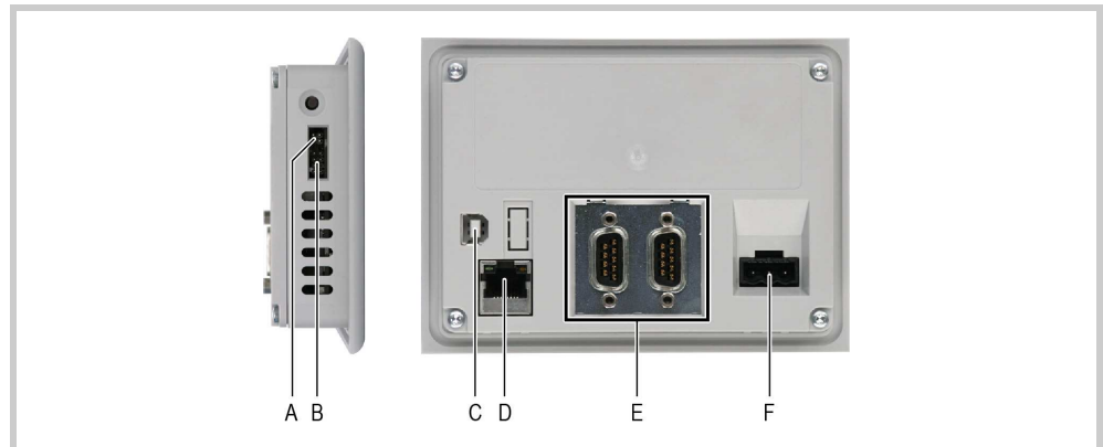
Abb. 6 Schnittstellen der 3,5"-Geräte
