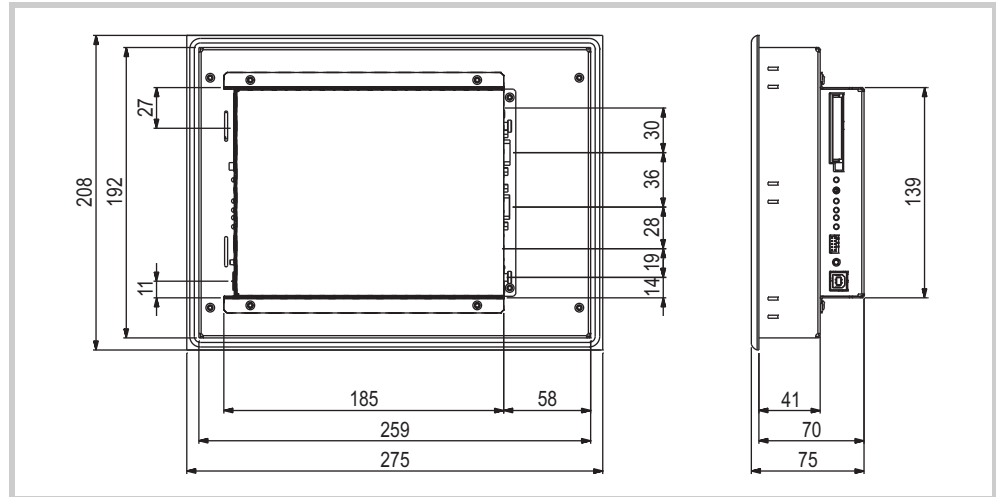
Abb. 29 Mechanische Abmessungen der 8,4"-Geräte in mm
