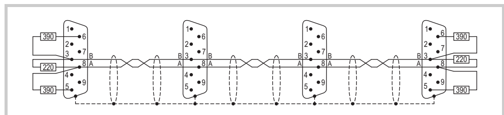
Abb. 19 Bussegment mit vier Busteilnehmern
