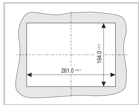
Abb. 21 Einbauausschnitt für 8,4"-Geräte
