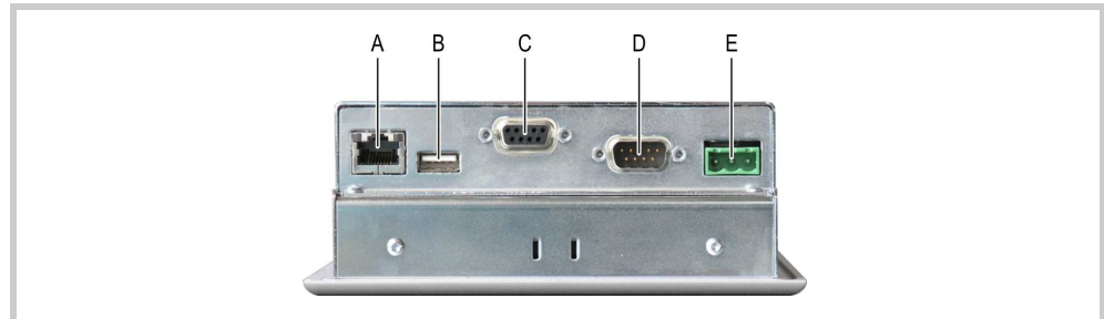
Abb. 8 Steckerseite des Geräts
