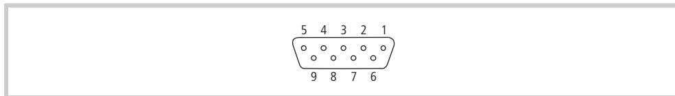
Abb. 18 Profibus-Schnittstelle (9-polig, D-Sub, female, UNC)
