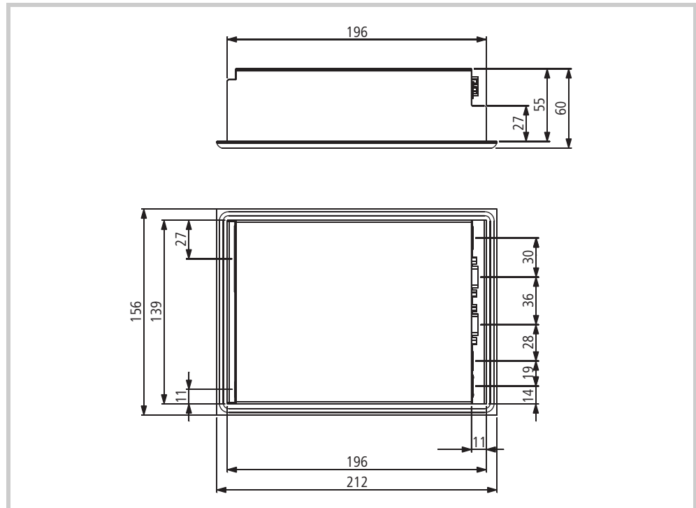
Abb. 28 Mechanische Abmessungen der 5,7"-Geräte in mm
