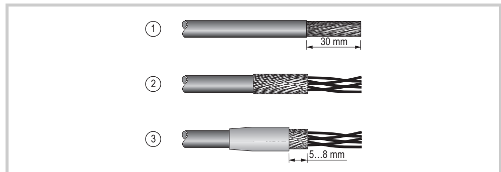
Abb. 10 Kabelschirm anschliessen
