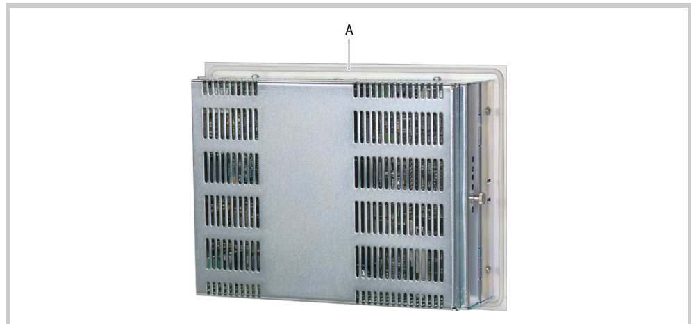
Abb. 22 Nut für Dichtungsschnur (A)
