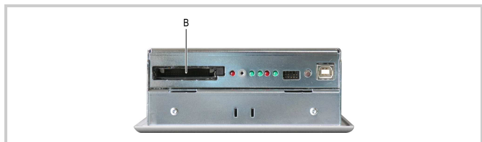
Abb. 27 Serviseite des Gerätes (CF-Slot-Abdeckung demontiert)
