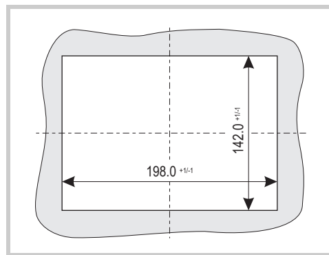
Abb. 20 Einbauausschnitt für 5,7"-Geräte
