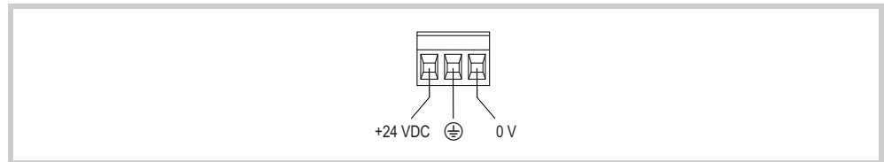
Abb. 13 Steckverbinder Phoenix Contact MSTB 2.5/3-ST-5.08 (Ansicht von der Verdrahtungsseite)
