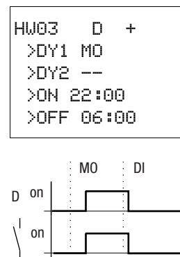
Abbildung 138:Wirkdiagramm „Nachtschaltung“
