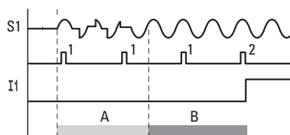
Abbildung 215: Taster, der prellt
