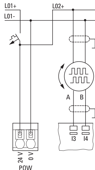
Abbildung 35: Inkrementalwertgeber an EASY806-DC-SWD
