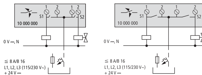
Abbildung 47: Relaisausgänge EASY2...-RE
