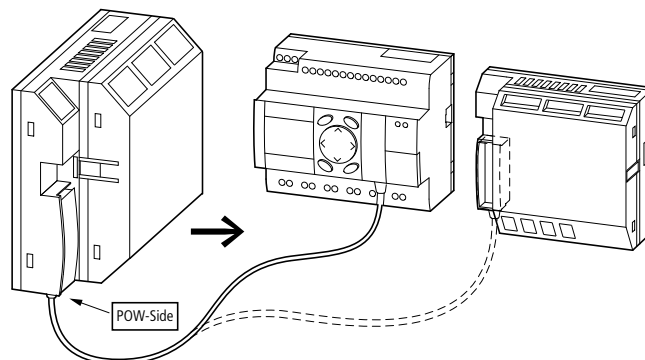
Abbildung 63: Punkt-zu-Punkt-Verbindung serielle Schnittstelle
