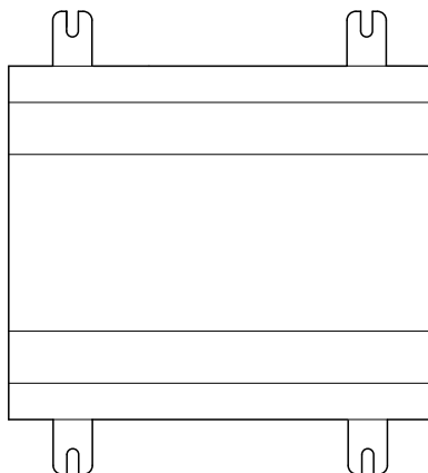
Abbildung 8: Schraubmontage easy800-Standard
