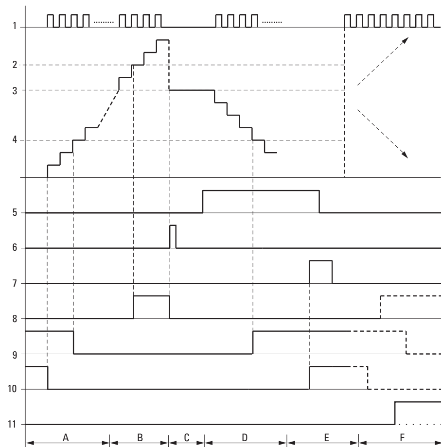
Abbildung 112: Wirkdiagramm Zählrelais
