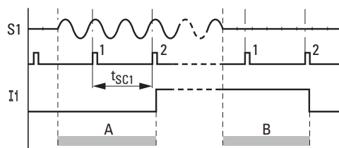
Abbildung 216: Schaltverhalten bei deaktivierter I-ENTPRELLUNG
