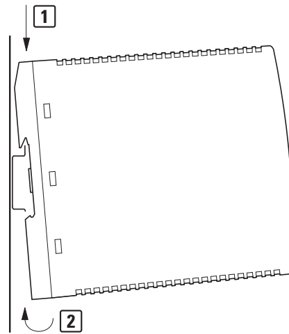
Abbildung 6: easy800-SWD
