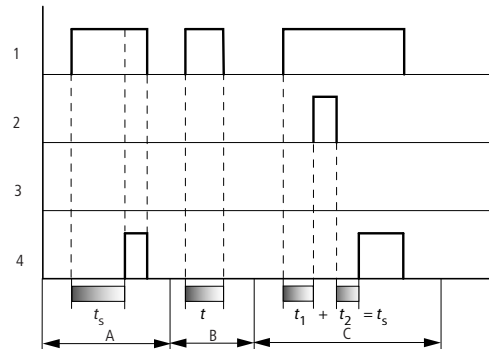
Abbildung 188: Wirkdiagramm Zeitrelais ansprechverzögert (mit/ohne Zufallsschalten)
