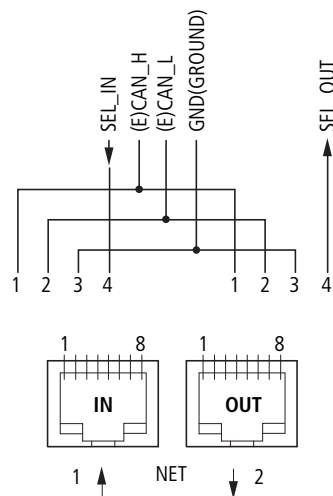
Abbildung 56: RJ45-Buchsen
