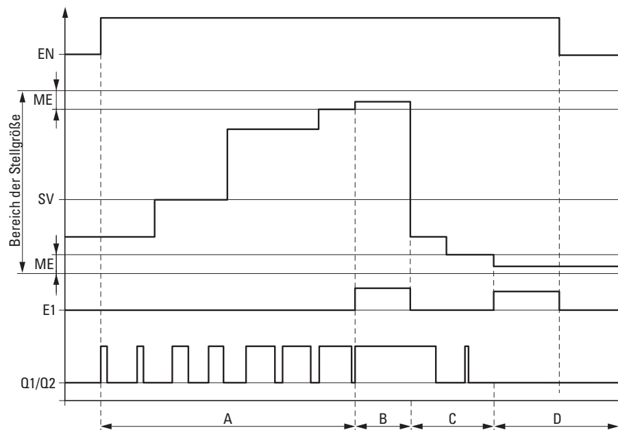
Abbildung 174: Wirkdiagramm Pulsweitenmodulation
