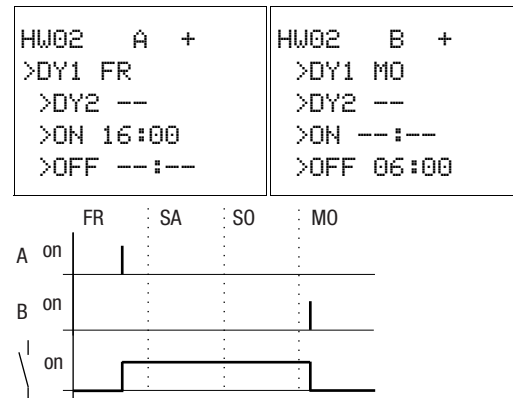
Abbildung 137:Wirkdiagramm „Wochenende“
