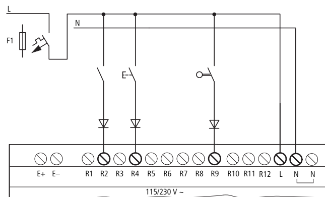
Abbildung 23: Eingänge beim AC-Erweiterungsgerät EASY618-AC-RE über Dioden anschließen
