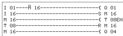
Abbildung 220: Automatischer Reset der Fehlermeldung
