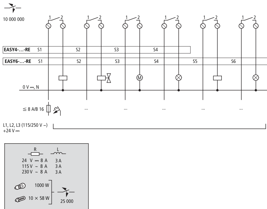
Abbildung 46: Relaisausgänge EASY4...-RE/EASY6...-RE.
