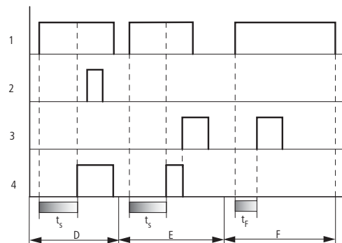
Abbildung 189: Wirkdiagramm Zeitrelais ansprechverzögert (mit/ohne Zufallsschalten)
