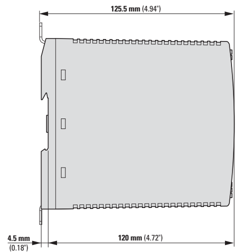
Abbildung 223: Abmessungen easy800-SWD
