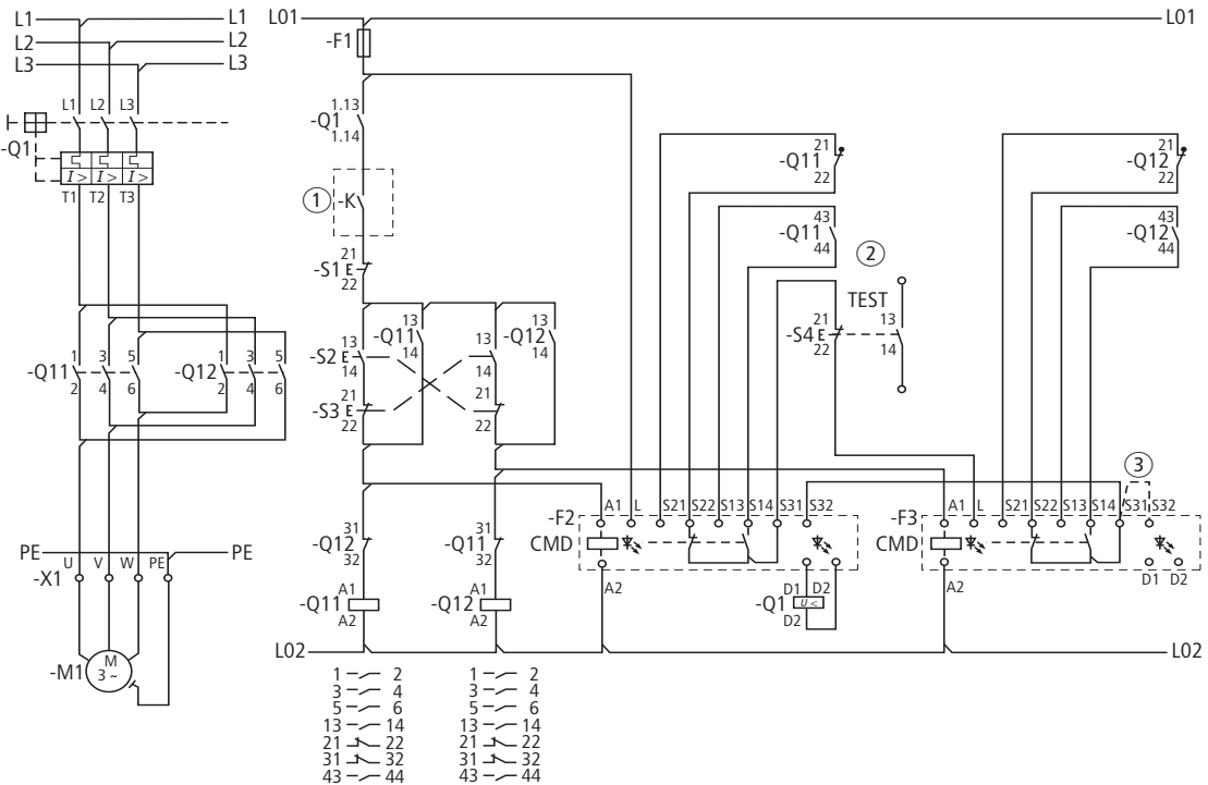
Figure 4 : Démarreur-inverseur
