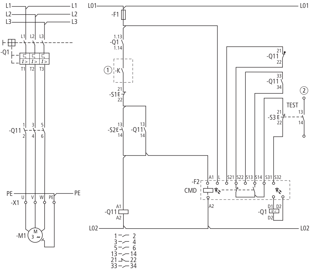
Figure 3 : Démarreur direct
