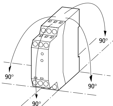
Figure 2 : Positions de montage pour CMD
