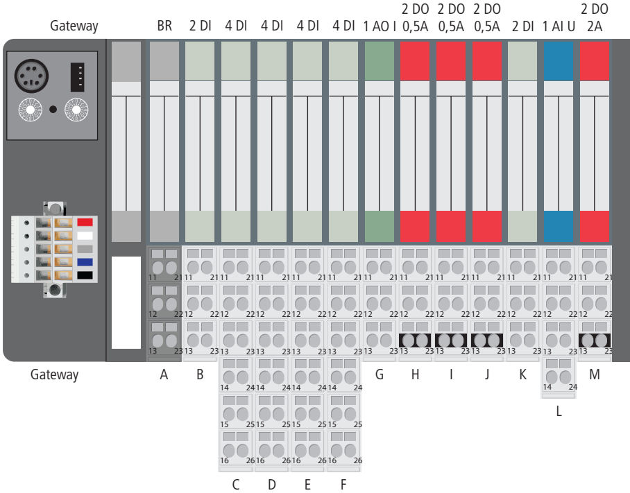
Abbildung 16: Beispielstation
