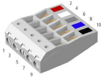
Abbildung 5: Open Style Connector (female / Oberseite)
