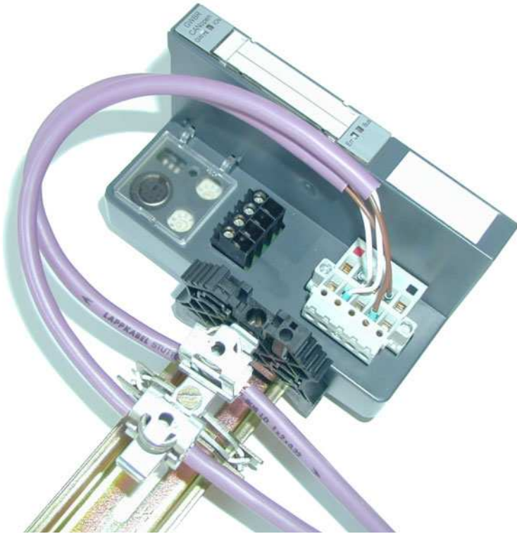
Abbildung 8: Schirmanschluss für ein XN-GWBR-DNET
