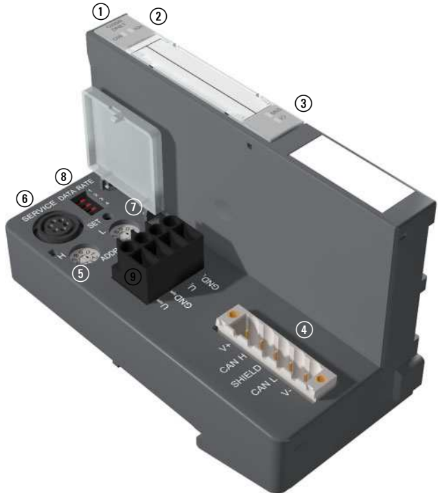
Abbildung 3: XN-GWBR-DNET
