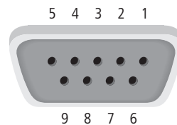
Abbildung 10: 9-polige SUB-D-Buchse am Anschlusskabel zum PC (Draufsicht)
