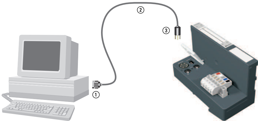
Abbildung 11: Verbindung zwischen PC und XI/ON-Gateway über das XI/ON-Verbindungskabel
