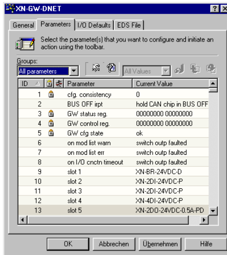
Abbildung 35: Stationsparameter
