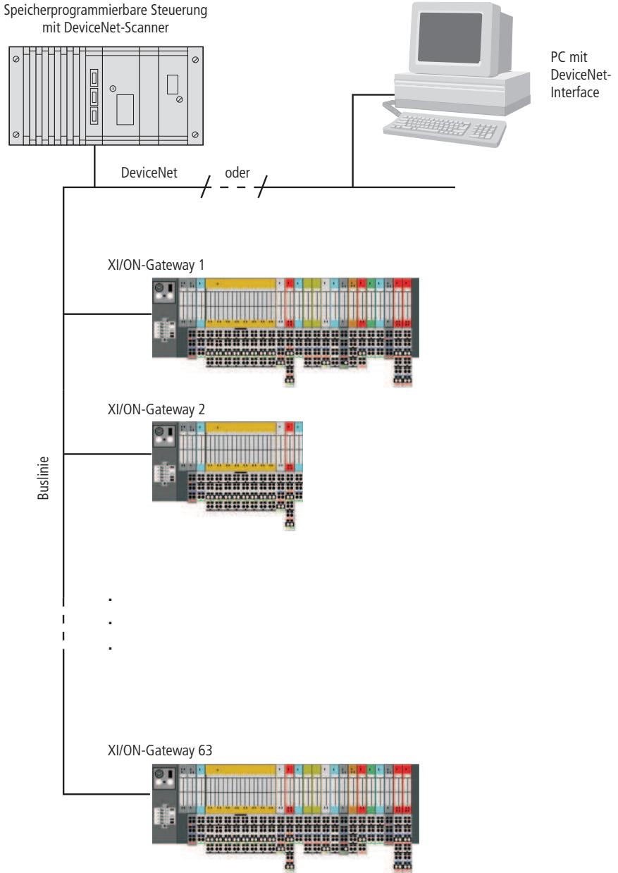
Abbildung 17: Maximaler Systemausbau
