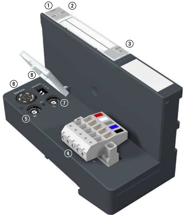
Abbildung 2: XN-GW-DNET
