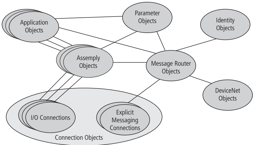
Abbildung 14: DeviceNet-Netzwerk
