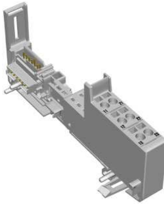
Abbildung 91: Basismodul XN-S3T-SBB
