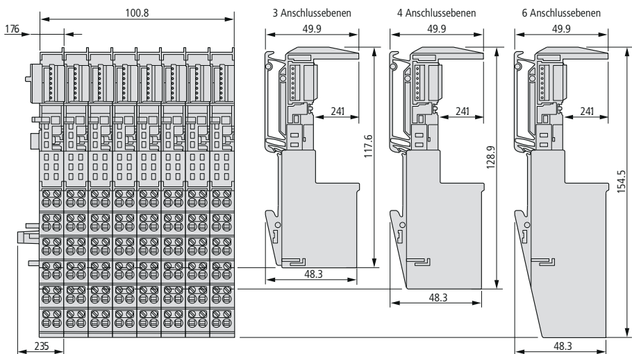
Abbildung 11: Basismodule in Blockausführung mit Schraubanschluss (XN-BxS...)
