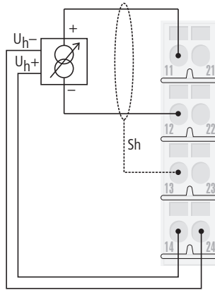
Abbildung 44: Anschlussbild XN-S4x-SBBS Analogwert- geber mit 2-Leiter Geberversorgung
