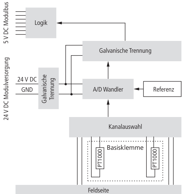
Abbildung 67: Blockschaltbild
