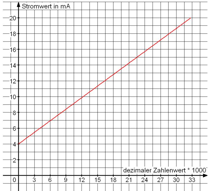
Abbildung 22: Darstellung der Stromwerte zu den dezimalen Werten im Koordinatensystem
