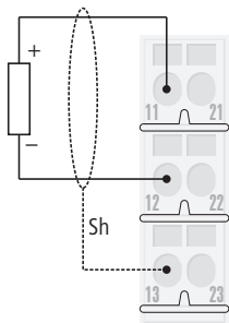
Abbildung 88: Anschlussbild XN-S3x-SBB
