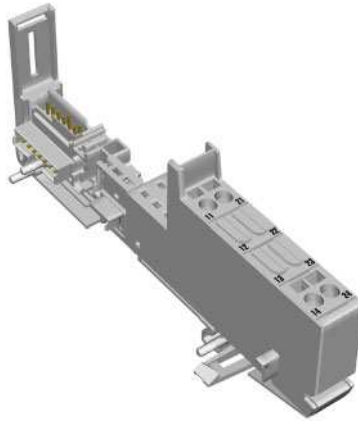
Abbildung 68: Basismodul XN-S4T-SBBS-CJ
