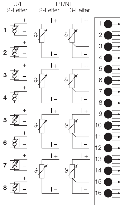
Abbildung 76: Anschlussmöglichkeiten
