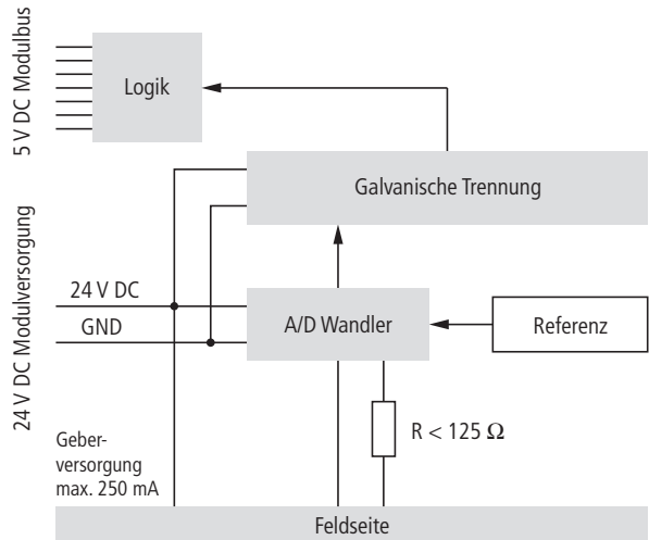
Abbildung 40: Blockschaltbild
