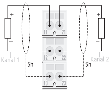
Abbildung 96: Anschlussbild XN-S3x-SBB
