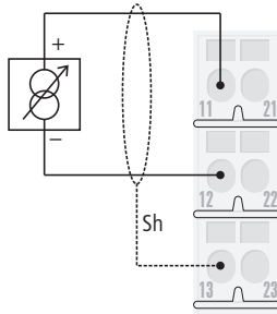
Abbildung 42: Anschlussbild XN-S3x-SBB Analogwert- geber ohne Gebersversorgung
