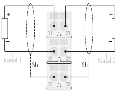
Abbildung 92: Anschlussbild XN-S3x-SBB
