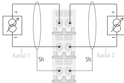
Abbildung 59: Anschlussbild XN-S3x-SBB
