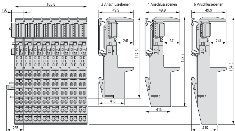
Abbildung 10: Basismodule in Blockausführung mit Zugfederanschluss (XN-BxT...)
