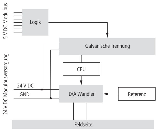
Abbildung 98: Blockschaltbild
