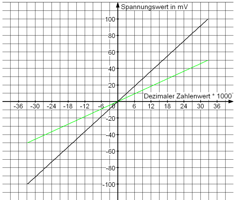
Abbildung 27: Darstellung der Spannungswerte zu den dezimalen Werten im Koordinatensystem für die Parametrierung " \pm 50\text{mV} " (grün) und " \pm 100\text{mV} " (schwarz)
