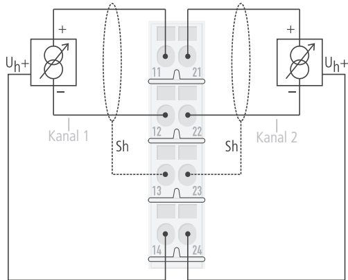
Abbildung 49: Anschlussbild XN-S4x-SBBS
