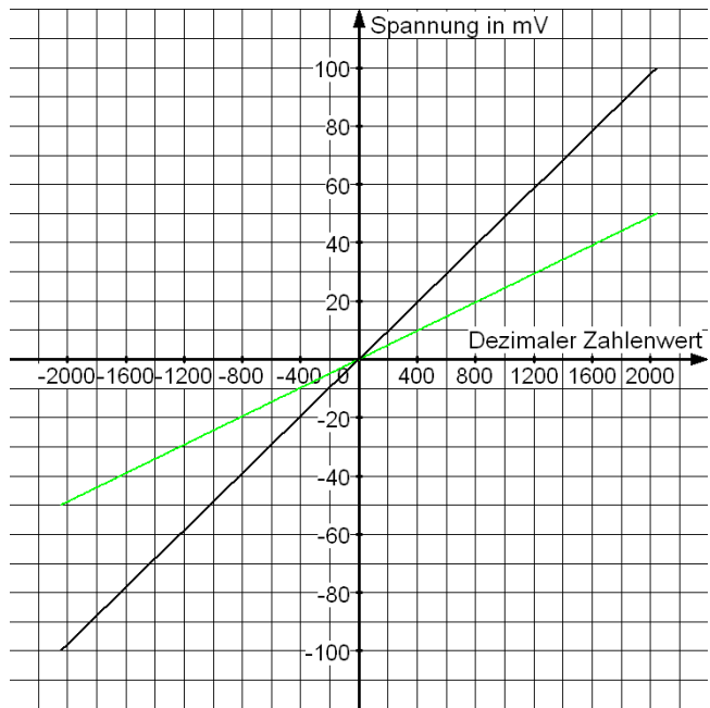
Abbildung 35: Darstellung der Spannungswerte zu den dezimalen Werten im Koordinatensystem für die Parametrierung " \pm 50\text{mV} " (grün) und " \pm 100\text{mV} " (schwarz)
