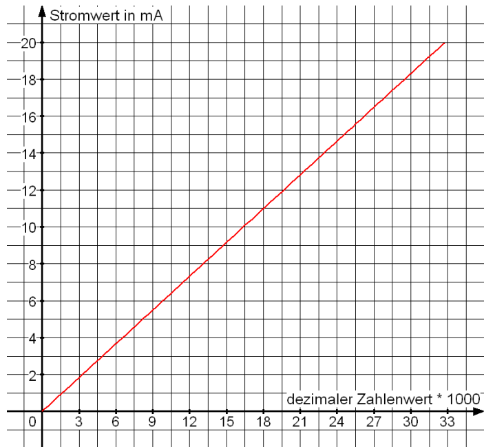
Abbildung 21: Darstellung der Stromwerte zu den dezipalcr Werten im Koordinatensystem
