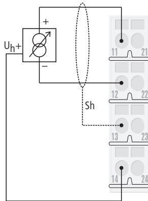
Abbildung 43: Anschlussbild XN-S4x-SBBS Analogwert- geber mit 1-Leiter Gebersversorgung
