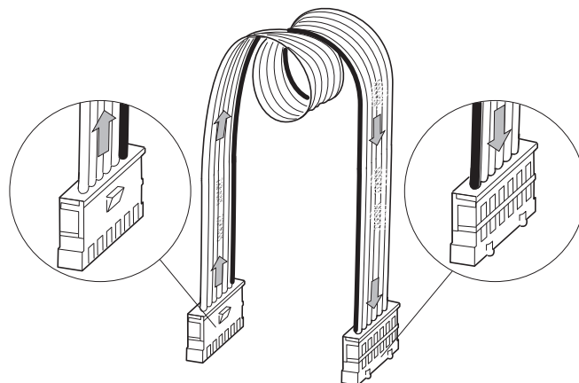
Abbildung 41: SWD-Flachleitung mit Flachstecker SWD4-8MF2 am Anfang und Ende
