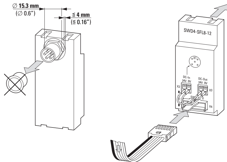
Abbildung 26: Schaltschrankdurchführung SWD4-SFL8-12
