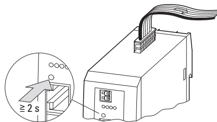
Abbildung 56: Konfigurationstaste am Gateway EU5C-SWD-DP
