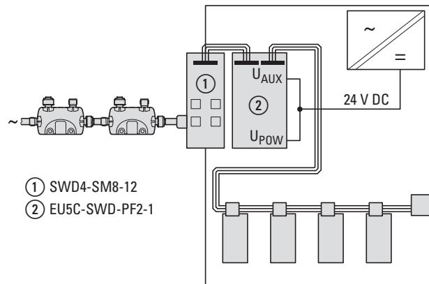
Abbildung 32: Spannungsversorgung über Powerfeed-Modul
