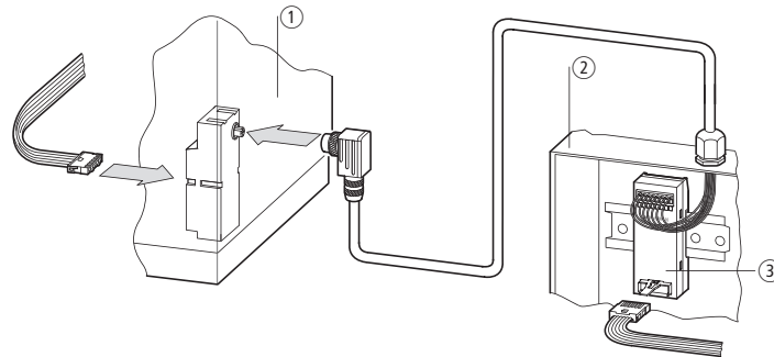
Abbildung 21: Beispiel für Übergang SWD-Flachleitung auf SWD-Rundleitung
