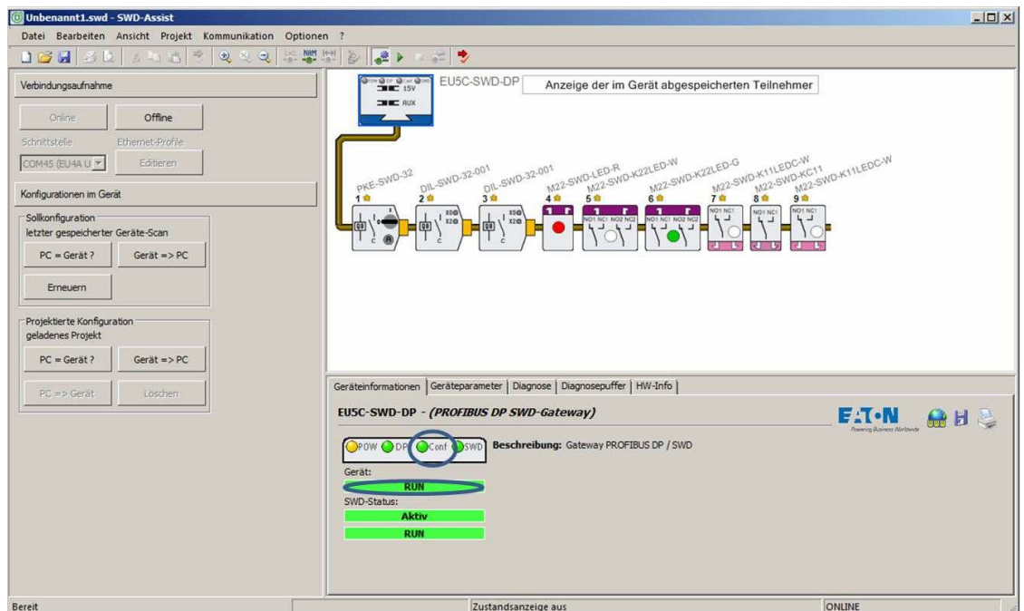
Abbildung 59: Überprüfen der Statusanzeige im Programm SWD-Assist nach erfolgreichem Laden der Projektkonfiguration
