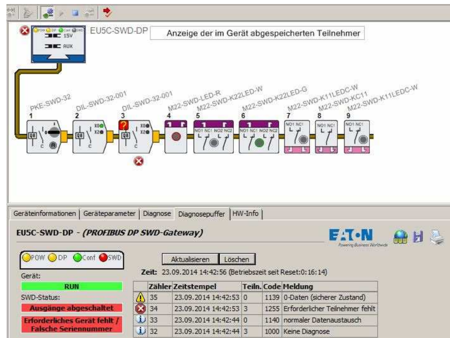
Abbildung 66: Anzeige eines fehlenden Teilnehmers in der Zustandsanzeige
