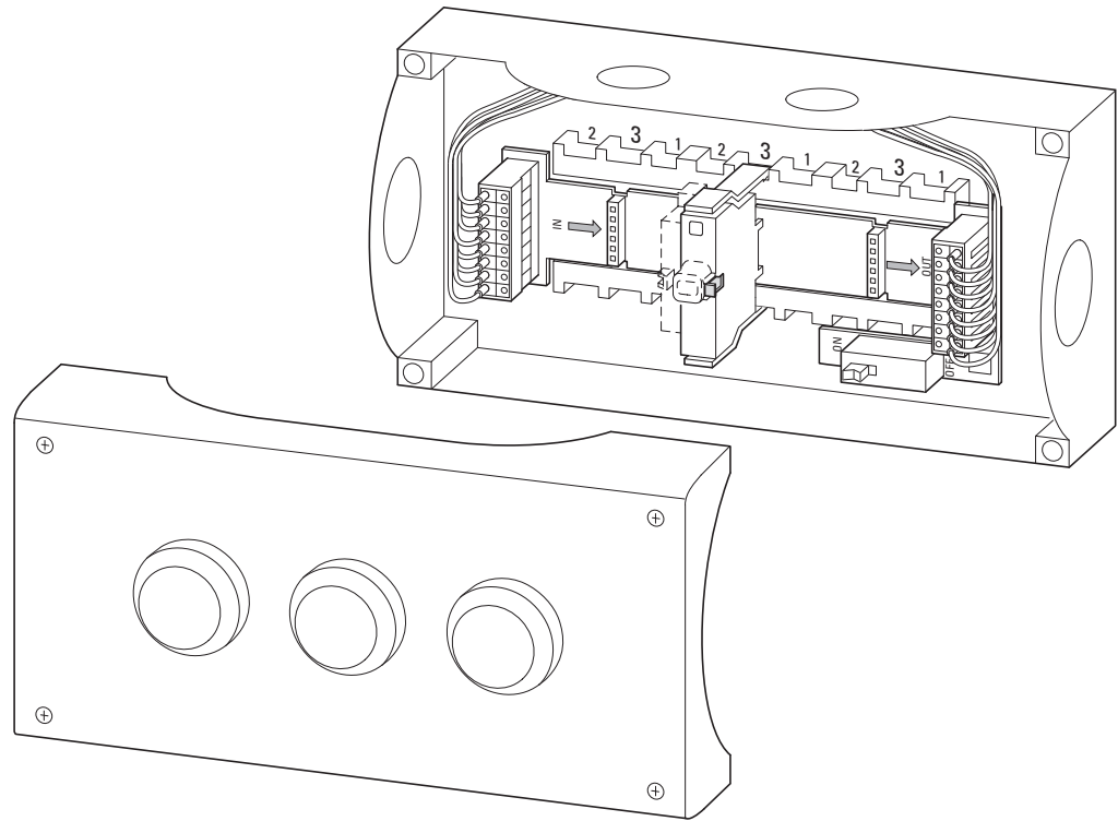
Abbildung 16: Leiterplatte in Aufbaugehäuse
