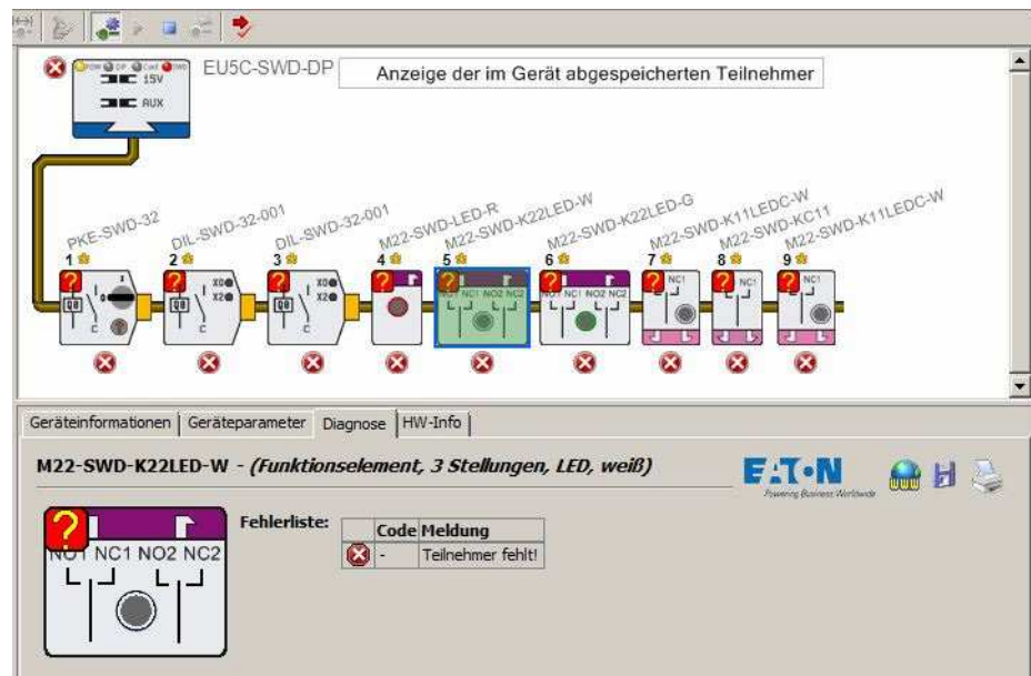
Abbildung 67: Keine Verbindung zwischen Koordinator und den SWD-Teilnehmern
