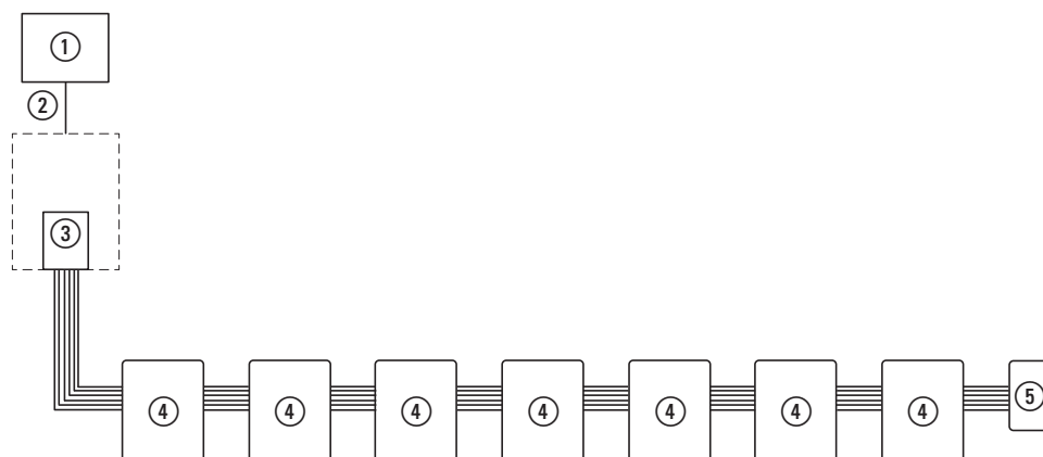
Abbildung 12: Koordinator mit SWD-Strang
