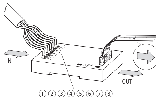
Abbildung 55: Adapter Flachstecker/Rundleitung mit Belegung des Federklemmenanschlusses
