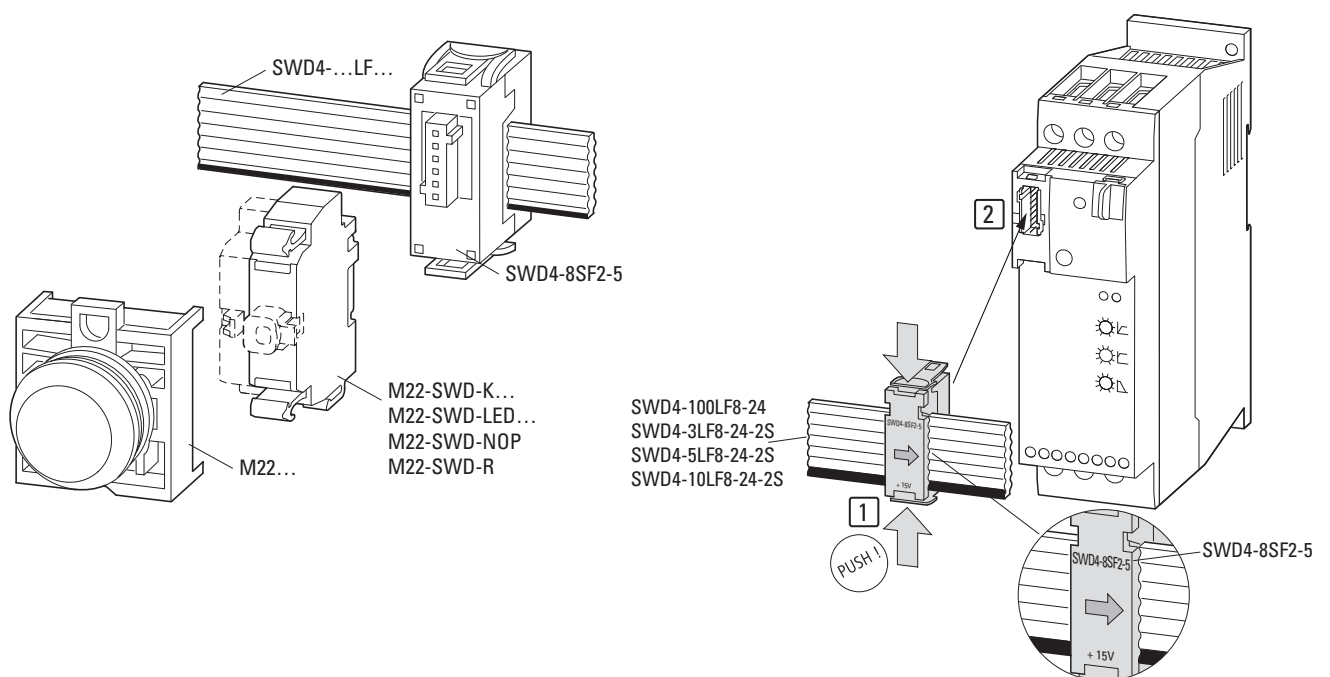
Abbildung 14: Beispiel: M22-SWD-Kommunikationsmodul (links), integrierte SWD-Lösung beim Softstarter DS7 (rechts)
