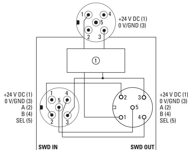
Abbildung 29: Einspeisen neuer Versorgungsspannung in der Peripherie mit dem Powerfeed-Modul EU5C-SWD-PF1
