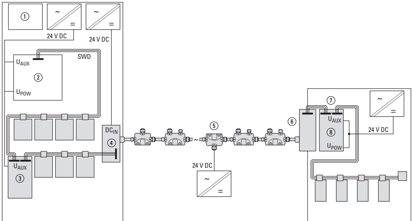
Abbildung 22: Beispiel zur Spannungsversorgung
