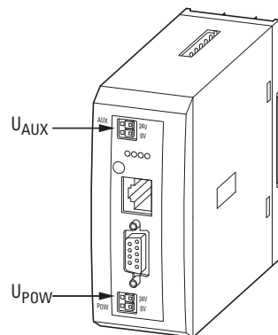
Abbildung 23: Spannungsversorgung am Gateway
