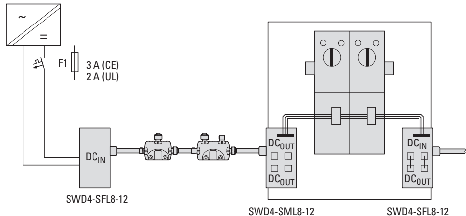
Abbildung 33: Strombegrenzung für die SWD-Flachleitung bei der Einspeisung auf die SWD-Rundleitung
