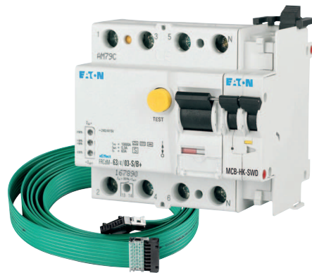
Abbildung 9: Sicherungshilfsschalter mit SmartWire-DT
