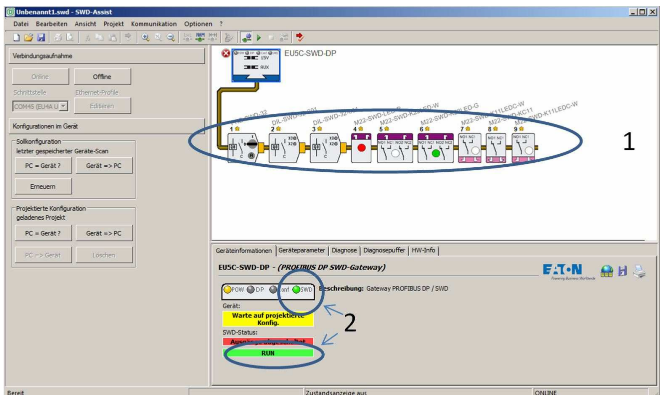
Abbildung 58: Anzeige der Soll-Konfiguration
