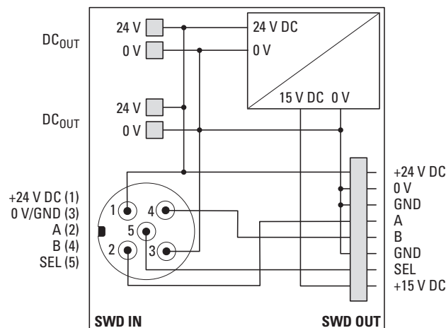
Abbildung 30: Schaltschrankdurchführung SWD4-SML8-12
