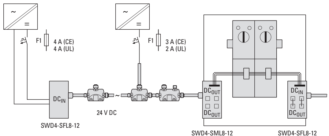
Abbildung 34: Strombegrenzung für die SWD-Flachleitung bei einer Einspeisung über ein Powerfeed-Modul EU1S-SWD-PF1-2
