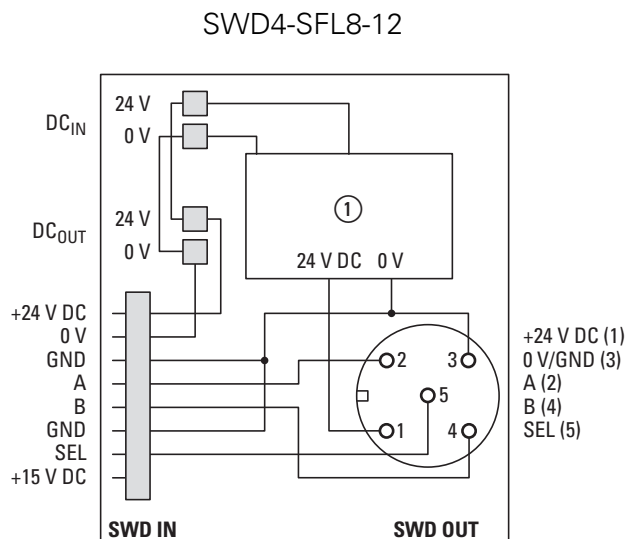
Abbildung 27: Verwendung der 24-V-DC-Spannung der SWD-Flachleitung zur Versorgung in der Peripherie
