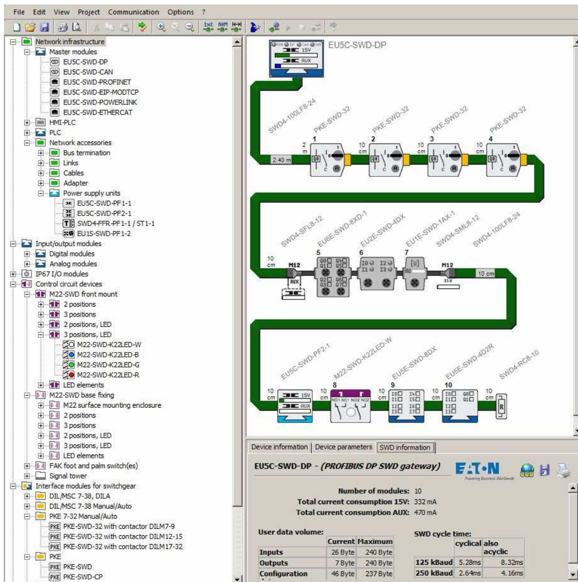
Abbildung 40: SmartWire-DT Planungs- und Bestellhilfe (SWD-Assist)
