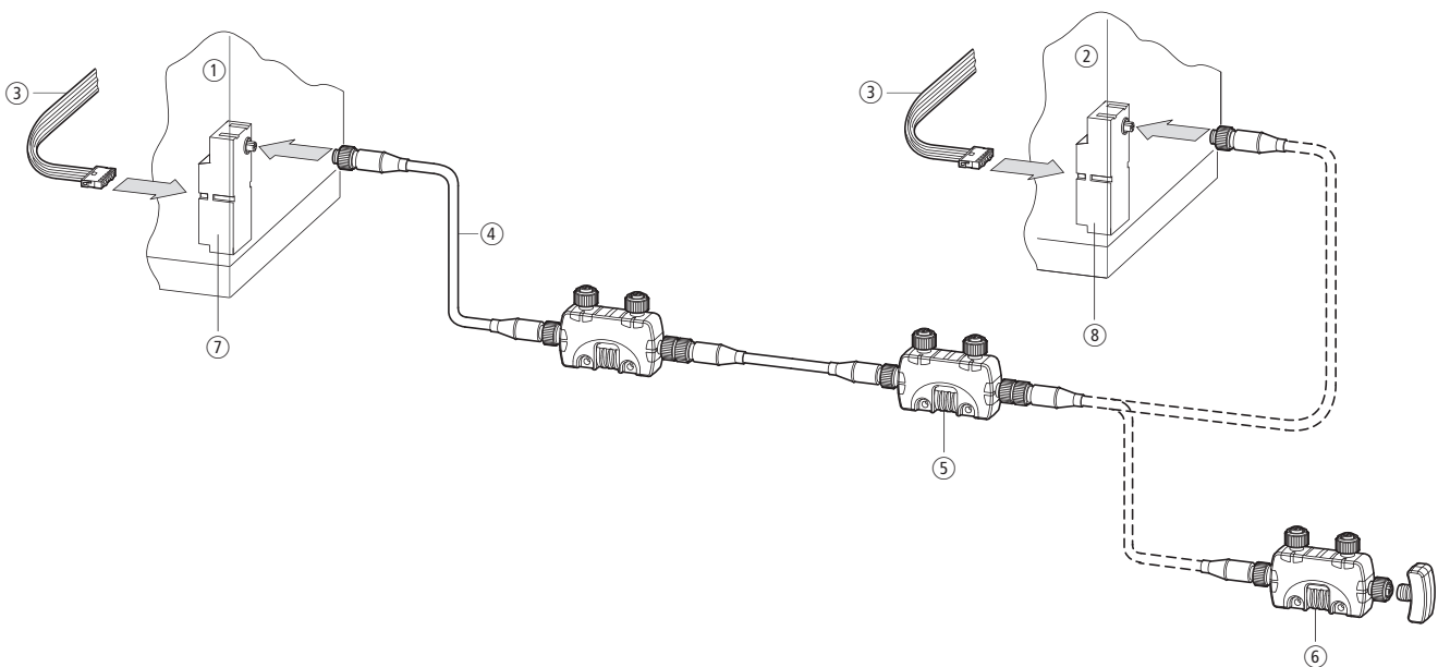
Abbildung 51: Leitungsadapter zum Übergang von der SWD-Flachleitung auf die SWD-Rundleitung und umgekehrt
