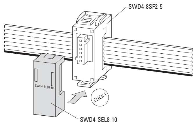
Abbildung 48: Brücke SWD4-SEL8-10 für Gerätestecker
