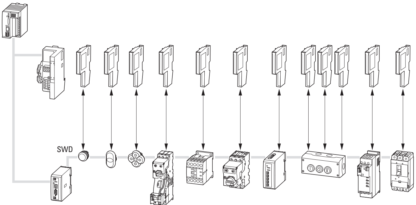
Abbildung 38: Gegenüberstellung einer Steuerungskonfiguration: Remote I/O (oben) – SmartWire-DT (unten)
