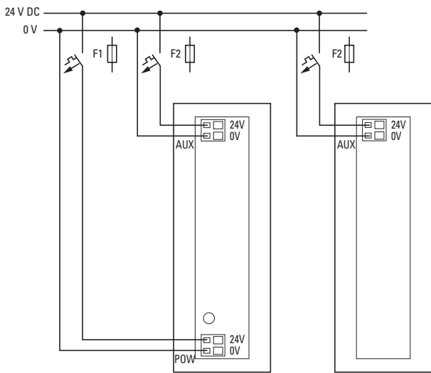
Abbildung 25: Spannungsversorgung Koordinator und Powerfeed-Module
