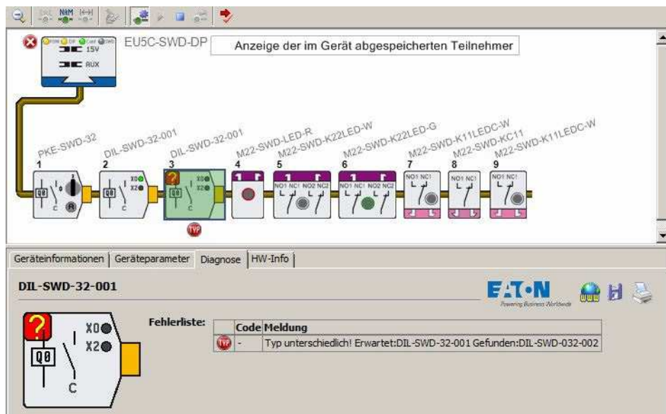
Abbildung 65: Anzeige eines falschen Geräts („unterschiedlicher Typ“) in der Zustandsanzeige
