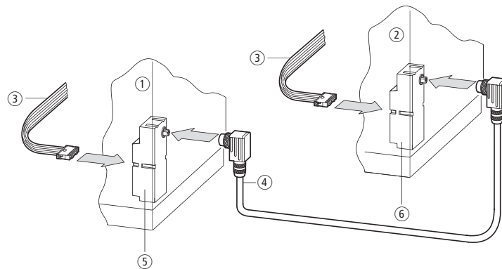
Abbildung 19: Schaltschrankdurchführung in Schaltschrank 1 als Rundbuchse, in Schaltschrank 2 als Rundstecker
