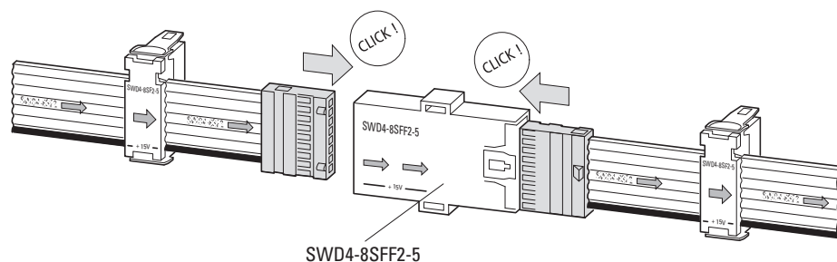
Abbildung 49: SWD-Flachleitungen mit Kupplung für 8-poligen Flachstecker verbinden
