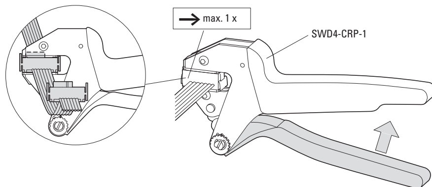
Abbildung 47: SWD-Gerätestecker in der Crimpzange verpressen
