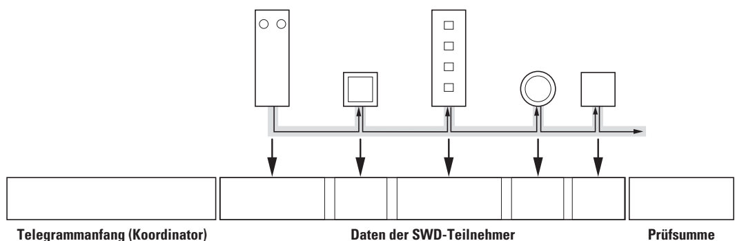
Abbildung 37: Telegrammaufbau
