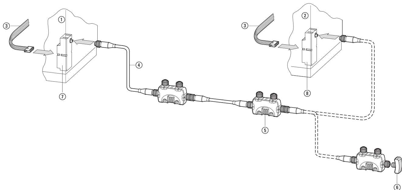
Abbildung 18: Übergang von Rund- auf Flachleitung
