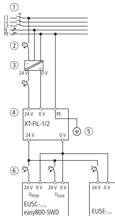
Abbildung 35: Spannungsversorgung mit EMV Filter
