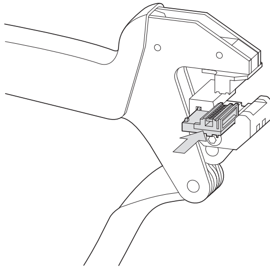
Abbildung 42: Flachstecker in die Crimpzange schieben
