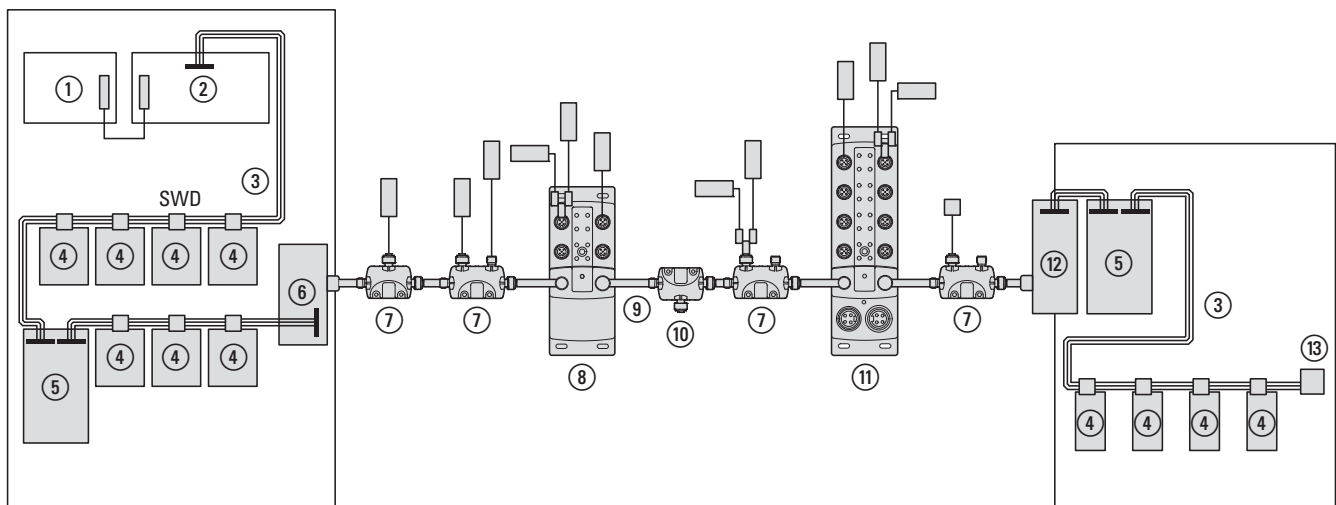
Abbildung 13: Flexible Netzwerkarchitektur in IP20 (Schaltschrank) und IP67 (Feld)
