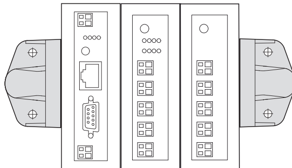
Abbildung 36: Montage mit zwei Stützwinkeln SL7/4-FW
