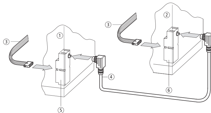
Abbildung 53: Schaltschrankdurchführung in Schaltschrank 1 als Rundbuchse, in Schaltschrank 2 als Rundstecker
