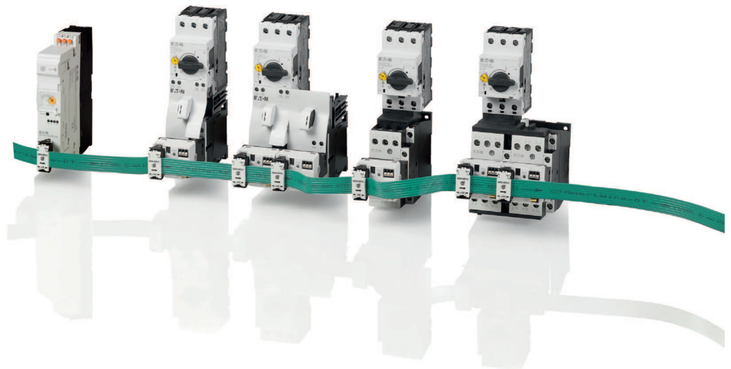
Abbildung 6: SmartWire-DT Anbindung für Schütze und Motorschutzschalter
