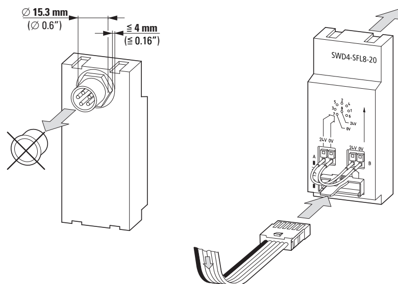
Abbildung 54: Leitungsadapter zum Übergang von SWD-Flach- auf 8-polige SWD-Rundleitung und umgekehrt SWD-Flachleitung
