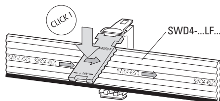
Abbildung 46: Gerätestecker montieren
