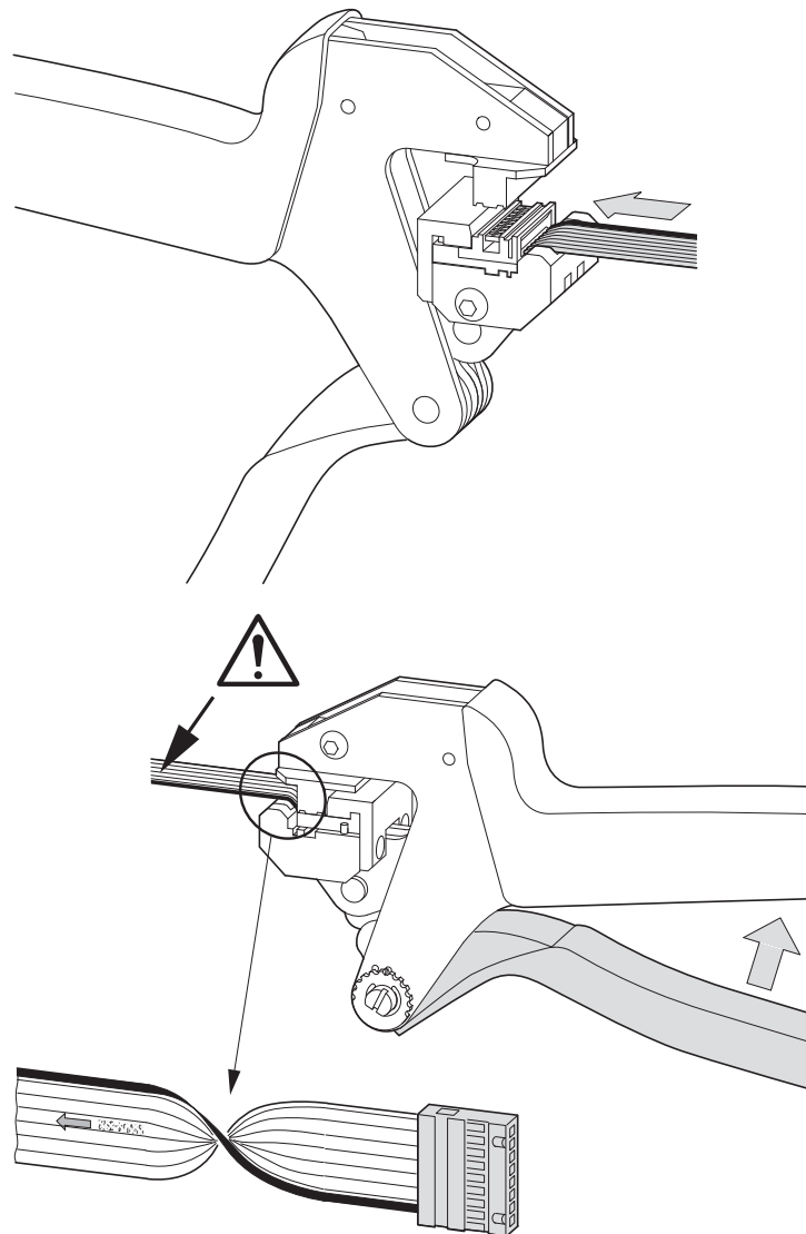
Abbildung 43: SWD-Flachleitung in Flachstecker schieben
