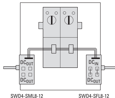
Abbildung 31: Beispiel: Anschluss von externen Motorschutzschaltern in der Peripherie
