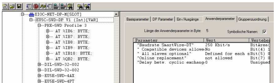
Abbildung 39: Parametrierung eines SWD-Netzwerks für ein PROFIBUS-DP-Netzwerk
