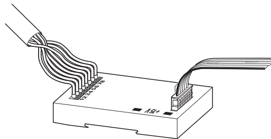
Abbildung 20: Leitungsadapter Flachstecker/Rundleitung
