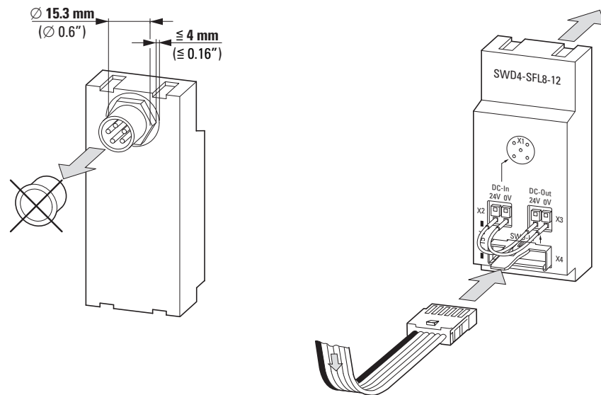
Abbildung 52: Schaltschrankdurchführung SWD4-SFL8-12
