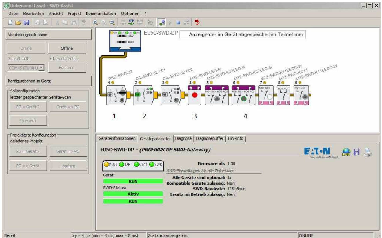
Abbildung 61: Zustandsanzeige im Programm SWD-Assist
