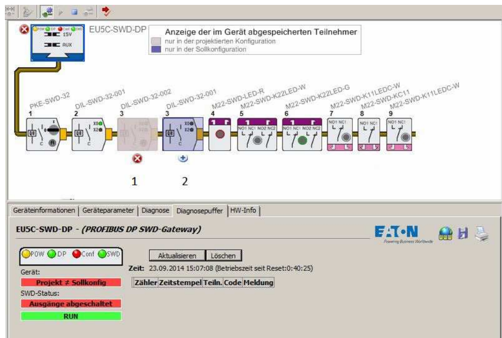
Abbildung 68: Abweichung zwischen Projekt- und Soll-Konfiguration
