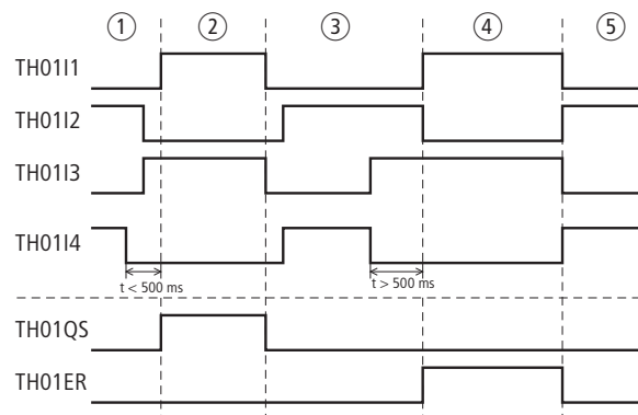
Abbildung 260: Beispiel 2 „Zweihandtaster“: Zeitdiagramm
