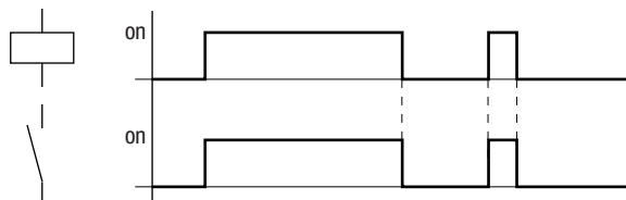
Abbildung 58: Wirkdiagramm „Schützfunktion“
