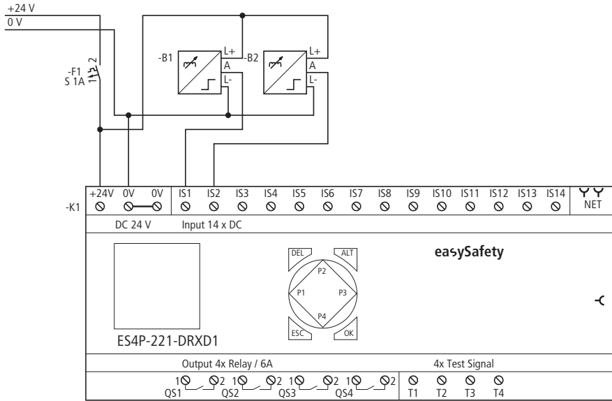
Abbildung 276:Beispiel „Stillstandsüberwachung“: Elektrischer Schaltplan
