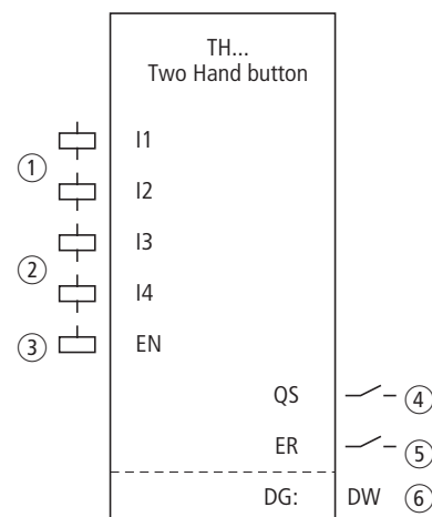
Abbildung 253:Funktionsbaustein „Zweihandtaster“
