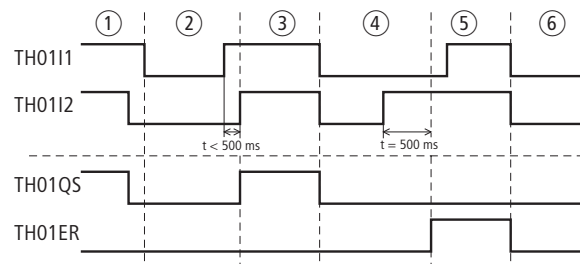
Abbildung 257:Beispiel 1 „Zweihandtaster“: Zeitdiagramm
