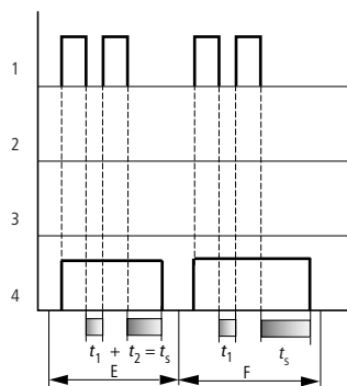
Abbildung 157: Wirkdiagramm Zeitrelais rückfallverzögert (mit/ohne Zufallsschalten, mit/ohne Retriggerung)
