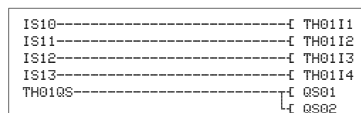
Abbildung 259: Beispiel 2 „Zweihandtaster“: Schaltplan in easySafety ES4P
