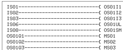
Abbildung 231: Beispiel „Betriebsartenwahlschalter“: Schaltplan in easySafety ES4P
