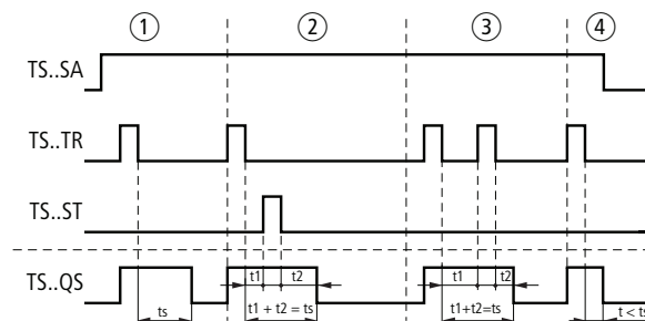
Abbildung 265:Wirkdiagramm „Zeitrelais rückfallverzögert“
