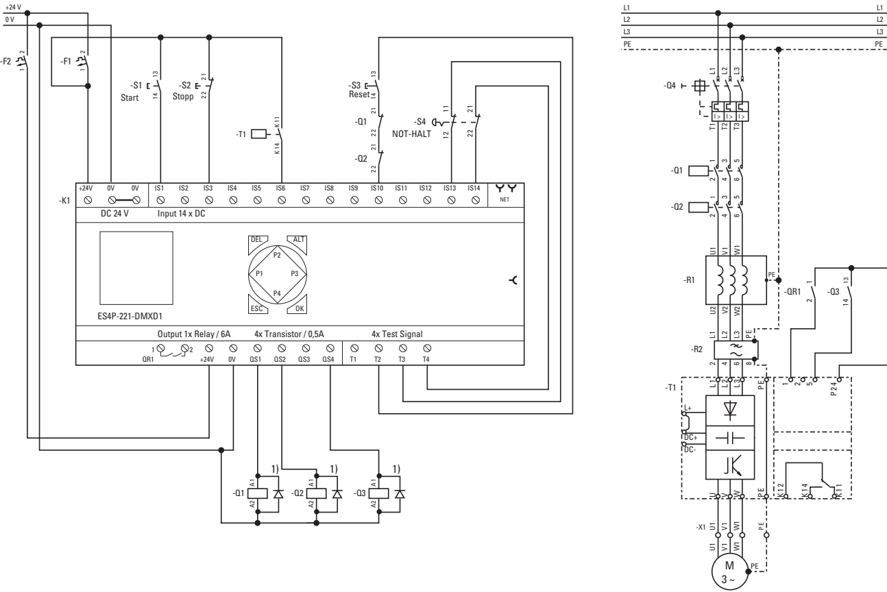
Abbildung 270: Beispiel, NOT-AUS: Elektrischer Schaltplan 1) Dioden-Löschglieder für Geräte ES4P-221-DMX.. der Geräteversionen 02 und 10 verwenden
