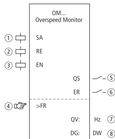
Abbildung 219:Funktionsbaustein „Höchstdrehzahlüberwachung“
