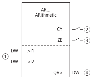
Abbildung 73: Funktionsbaustein „Arithmetik“
