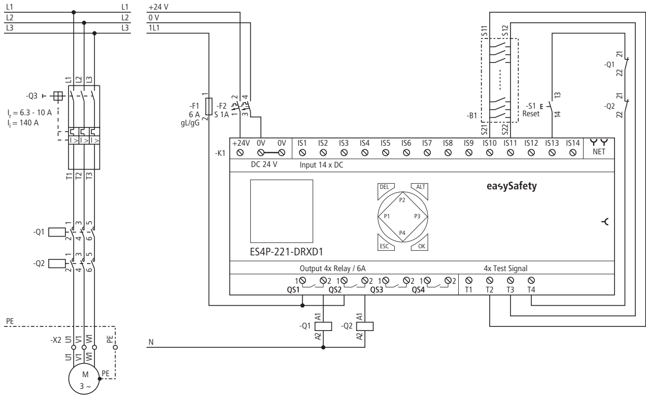
Abbildung 250: Beispiel „Schaltmatte“: Elektrischer Schaltplan
