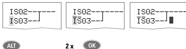
Abbildung 50: Kontakt I503 von Schließer zu Öffner ändern
