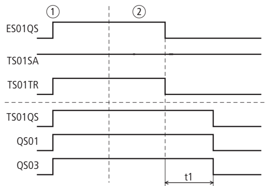
Abbildung 272: Beispiel 2 NOT-AUS: Zeitdiagramm
