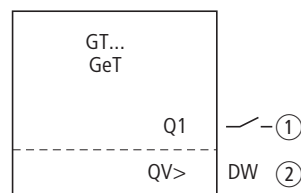
Abbildung 101:Funktionsbaustein GT
