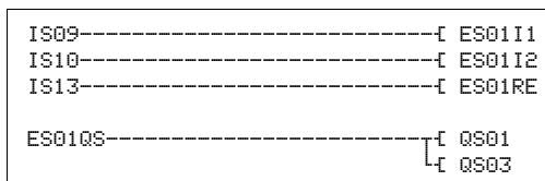
Abbildung 298:Schaltplan in easySafety
