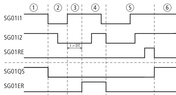
Abbildung 243: Beispiel 1 „Schutztür“: Zeitdiagramm
