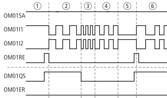
Abbildung 225: Beispiel „Höchstzahlüberwachung“: Zeitdiagramm
