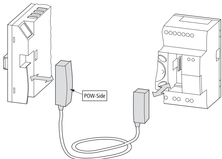
Abbildung 27: Verbindungsstecker stecken: links MFD-CP..., rechts easySafety ES4P
