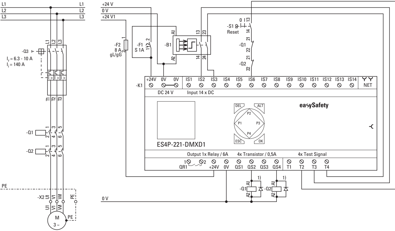
Abbildung 204: Beispiel 2 „Lichtgitter“: Elektrischer Schaltplan 1) Dioden-Löschglieder für Geräte ES4P-221-DMX.. der Geräteversionen 02 und 10 verwenden
