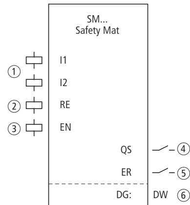
Abbildung 247: Funktionsbaustein „Schutztürüberwachung“
