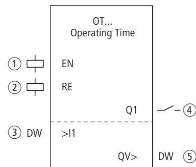
Abbildung 132: Funktionsbaustein „Betriebsstundenzähler“
