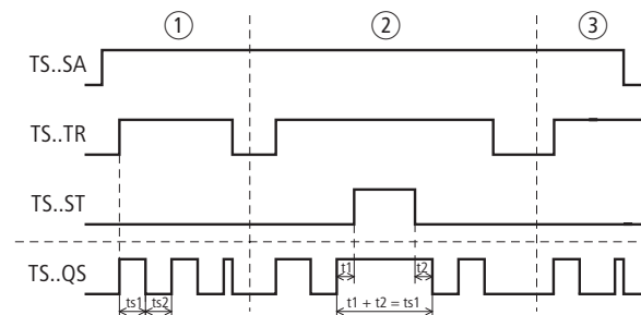
Abbildung 269: Wirkdiagramm „Zeitrelais, blinkend synchron und asynchron“
