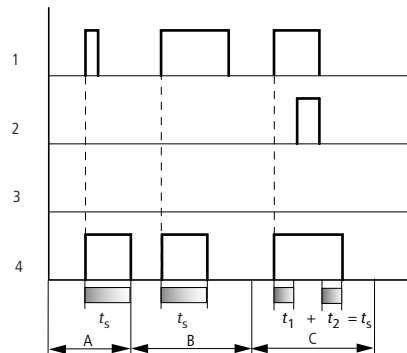
Abbildung 161: Wirkdiagramm Zeitrelais, Impulsformend 1
