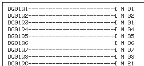
Abbildung 100: Verdrahtung der Ausgangskontakte
