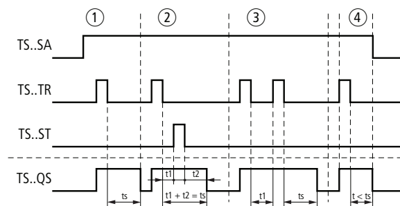
Abbildung 266: Wirkelement „Zeitrelais rückfallverzögert“ (mit/ohne Retriggerung)
