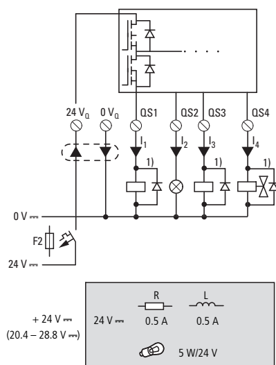
Abbildung 18: Transistor-Ausgänge ES4P-22.-DM..
