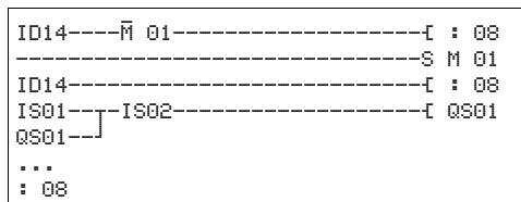
Abbildung 300:Standard-Schaltplan zum Überprüfen der Erweiterung
