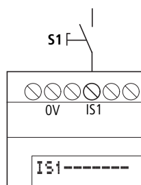
Abbildung 295: easySafety ES4P-Eingang mit Schalter belegt
