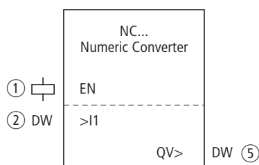
Abbildung 130:Funktionsbaustein „Zahlenwandler“
