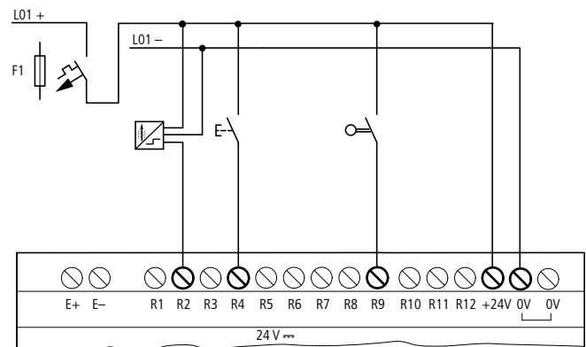
Abbildung 12: EASY6...-DC-.E (Standard-Erweiterungsgerät)
