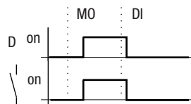
Abbildung 107:Wirkdiagramm „Nachtschaltung“
