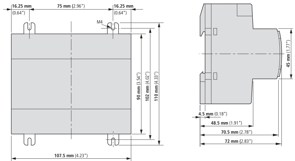
Abbildung 301: Abmessungen easySafety ES4P in mm (Angaben in inches → Tabelle 38)
