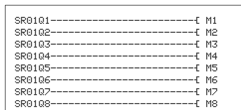
Abbildung 144: Betriebsart BIT, Verdrahtung der Bausteinkontakte
