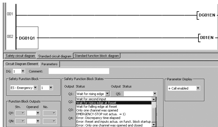
Abbildung 299: Zuordnung von Diagnose- und Sicherheits-Funktionsbaustein mit easySoft-Safety
