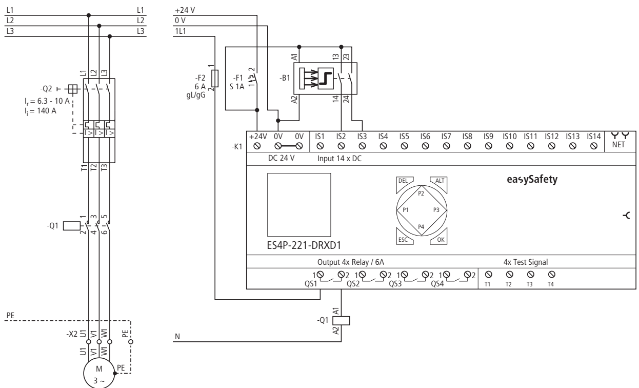
Abbildung 201:Beispiel 1 „Lichtgitter“: Elektrischer Schaltplan
