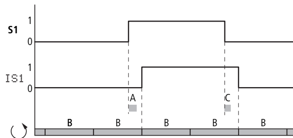
Abbildung 297: Schaltverhalten bei deaktivierter I-ENTPRELLUNG
