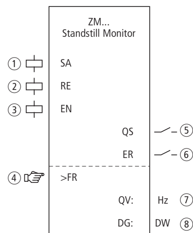
Abbildung 273: Funktionsbaustein „Stillstandsüberwachung“
