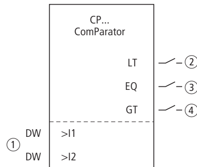
Abbildung 87: Funktionsbaustein „Vergleicher“
