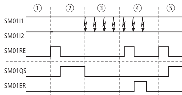
Abbildung 252:Beispiel „Schaltmatte“: Zeitdiagramm
