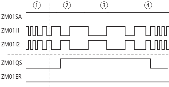
Abbildung 278:Beispiel „Stillstandsüberwachung“: Zeitdiagramm
