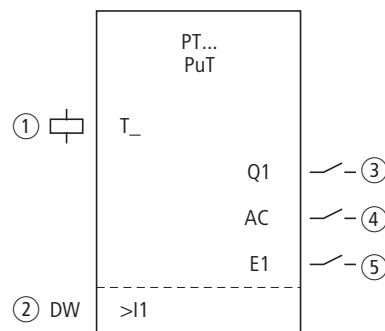
Abbildung 135:Funktionsbaustein PUT
