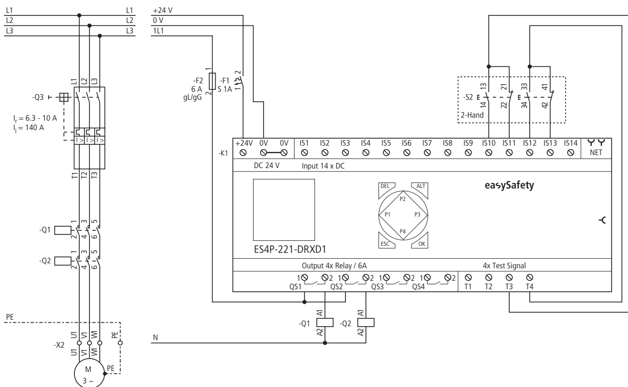
Abbildung 258: Beispiel 2 „Zweihandtaster“: Elektrischer Schaltplan
