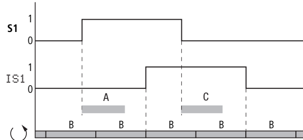
Abbildung 296: Verzögerungszeiten bei der Auswertung eines Eingangssignales und aktivierter I-ENTPRELLUNG
