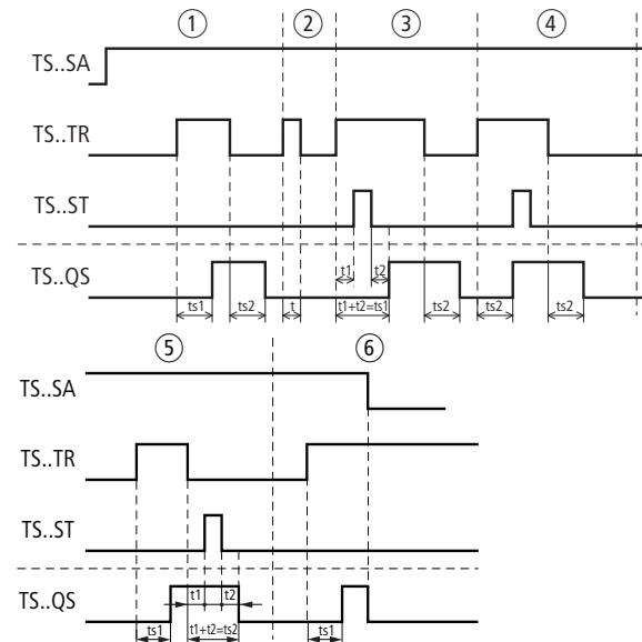
Abbildung 267: Wirksamdiagramm „Zeitrelais, ansprech- und rückfallverzögert“
