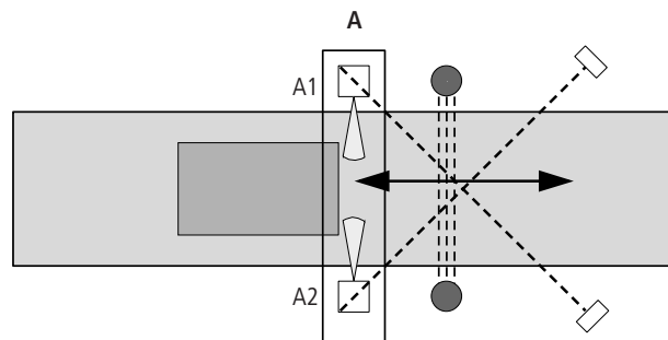
Abbildung 215: Lichtgitter Muting: Paralleles Muting mit 2 Mutingsensoren
