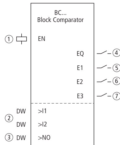
Abbildung 75: Funktionsbaustein „Datenblock-Vergleicher“
