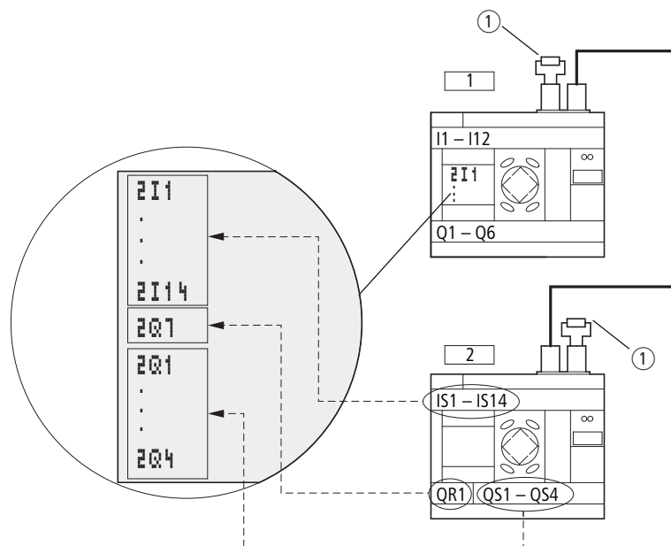
Abbildung 286: Ein- und Ausgänge eines easySafety ES4P-Gerätes im Standard-Schaltplan eines anderen Teilnehmers verwenden
