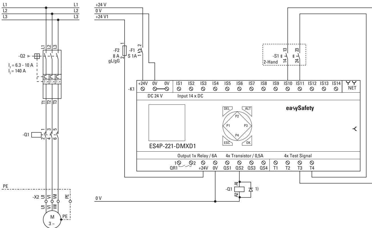
Abbildung 256: Beispiel 1 „Zweihandtaster“: Elektrischer Schaltplan
