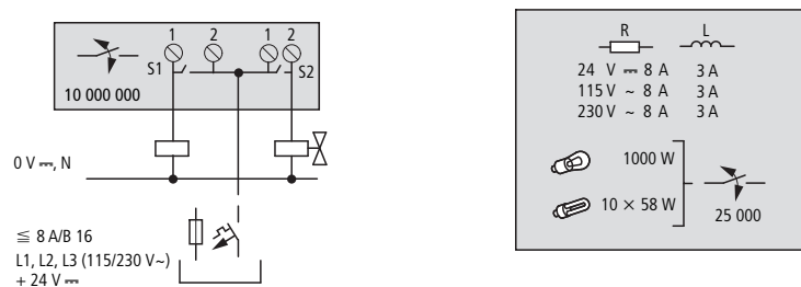
Abbildung 17: Relais-Ausgänge EASY2...-RE..
