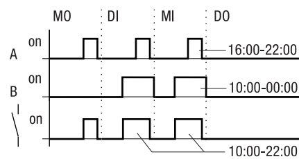
Abbildung 108:Wirkdiagramm Überschneidungen
