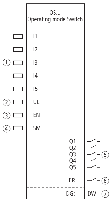
Abbildung 227: Funktionsbaustein „Betriebsartenwahlschalter“
