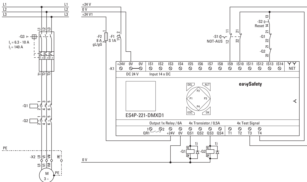
Abbildung 187: Beispiel NOT-AUS: Elektrischer Schaltplan
