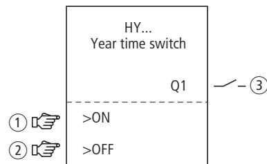
Abbildung 109:Funktionsbaustein „Jahresschaltuhren“
