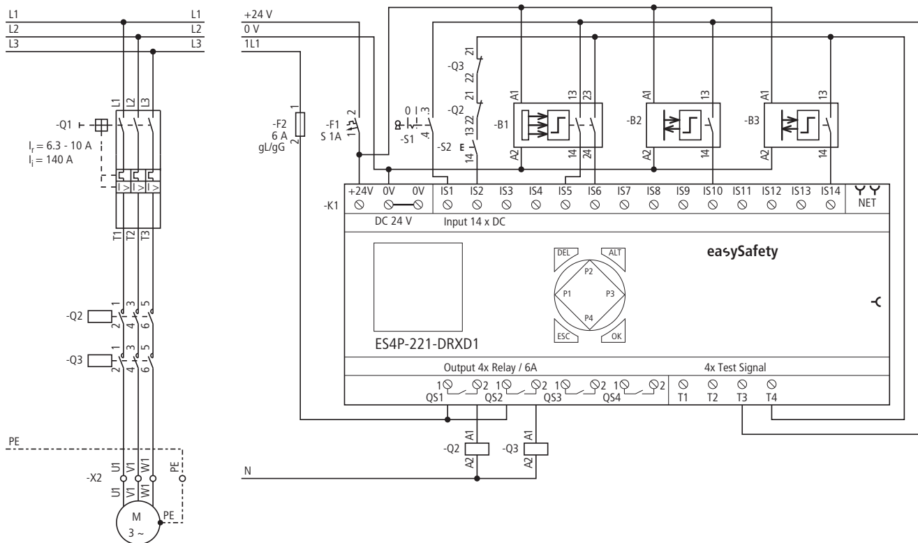
Abbildung 216: Beispiel „Lichtgitter Muting“: Elektrischer Schaltplan
