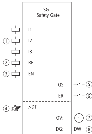
Abbildung 238:Funktionsbaustein „Schutztür“
