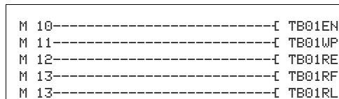
Abbildung 165: Verdrahtung der Bausteinspulen
