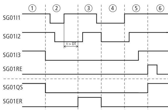
Abbildung 246: Beispiel 2 „Schutztür“: Zeitdiagramm
