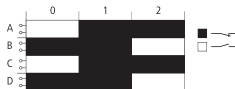
Abbildung 194: Kontaktgabe des 4-kanaligen Fußschalters mit drei Stufen 0, 1, 2 und vier Kontakten A, B, C, D
