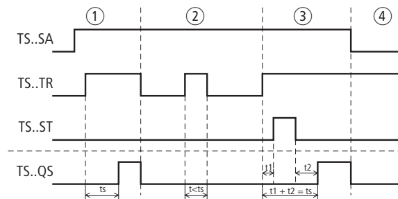
Abbildung 264:Wirkdiagramm „Zeitrelais ansprechverzögert“
