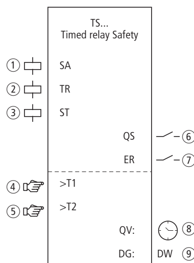
Abbildung 261:Funktionsbaustein „Zeitrelais“
