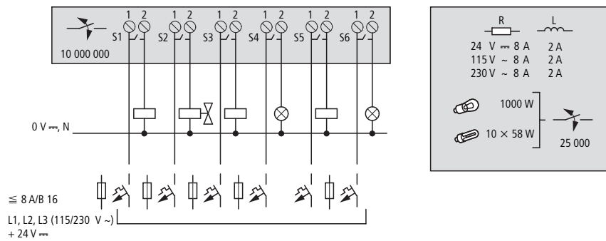
Abbildung 16: Relais-Ausgänge EASY6...-RE..
