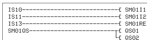
Abbildung 251: Beispiel 1 „Schaltmatte“: Schaltplan in easySafety ES4P
