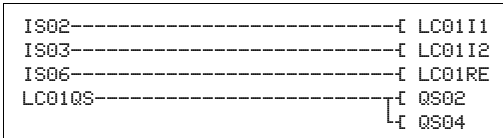
Abbildung 205: Beispiel 2 „Lichtgitter“: Schaltplan in easySafety ES4P
