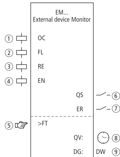
Abbildung 171: Funktionsbaustein „Rückführkreisüberwachung“
