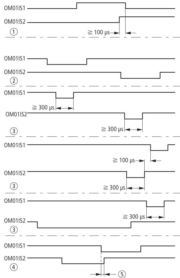
Abbildung 226: Zeitliches Verhalten der Signale an IS1/IS2
