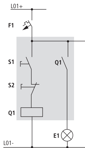
Abbildung 33: Lampensteuerung mittels Relais
