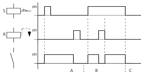
Abbildung 60: Wirkdiagramm „Setzen“ und „Rücksetzen“
