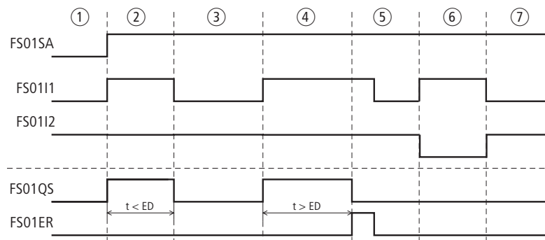
Abbildung 197: Beispiel „Fußschalter“: Zeitdiagramm
