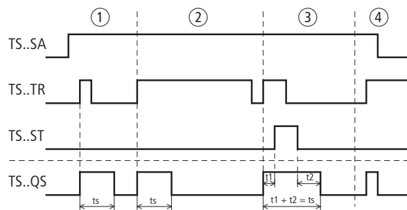
Abbildung 268: Wirkdiagramm „Zeitrelais, impulsformend“
