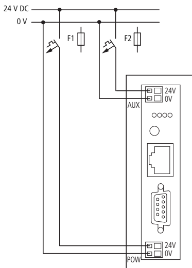
Figura 2: Collegamento
