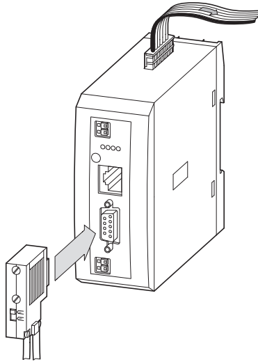
Figura 7: Collegamento di PROFIBUS-DP
