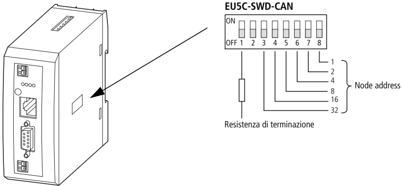
Figura 34: Attivazione della resistenza di terminazione
