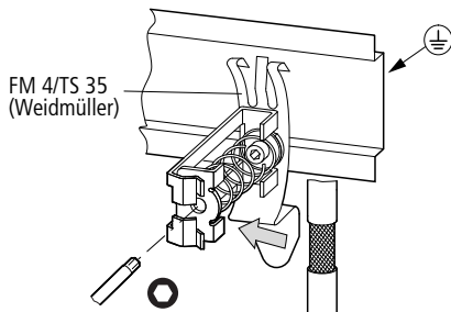
Figura 35: Schermatura della linea di rete
