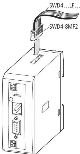
Figura 33: Collegamento SmartWire-Darwin
