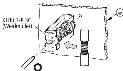
Figura 35: Schermatura della linea di rete
