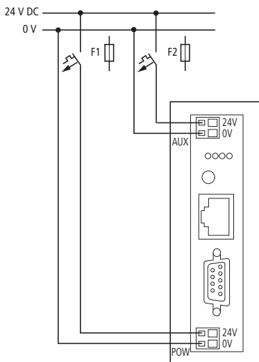
Figura 29: Collegamento
