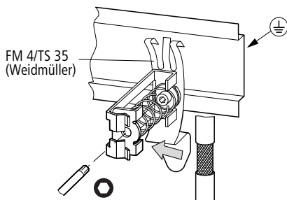
Figura 8: Schermatura della linea di rete
