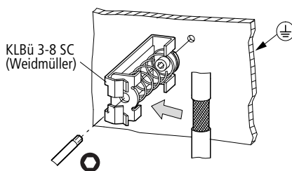
Figura 8: Schermatura della linea di rete
