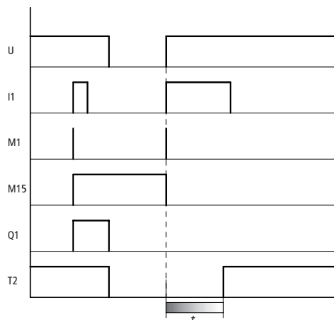
Diagramme dynamique :
