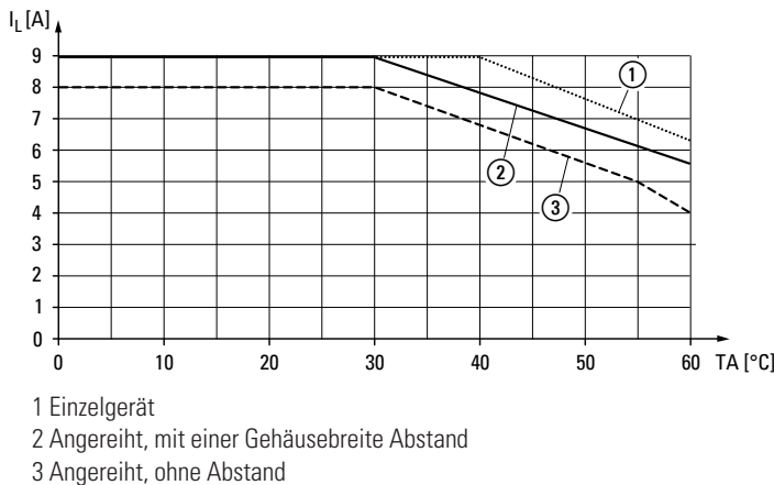
Bemessungsbetriebsstrom EMS-...-9-...
