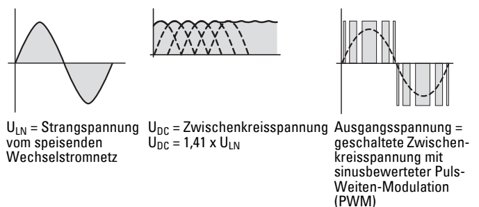
Blockschaltbild mit Hauptkomponenten eines Frequenzumrichters
