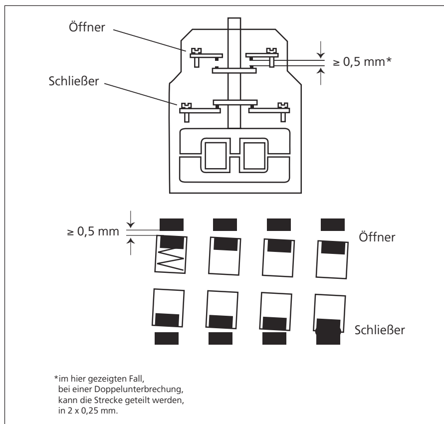
Bild 2: Wenn bei einem Schütz z.B. der rechts außen liegende Schließerkontakt verschweißt, kann sich die Kontaktbrücke des ausgeschalteten Schützes etwas schief stellen. Bei „zwangsgeführten Kontakten“ wird verlangt, dass in diesem Fall die Öffner nicht schliessen dürfen, sondern, dass über die gesamte Lebensdauer des Schützes ein Kontaktabstand von mindestens 0,5 mm erhalten bleibt. Verschiedene Sicherheitsschaltungen basieren auf der Voraussetzung, das Öffner und Schließer eines Schützes niemals gleichzeitig geschlossen sein können.
