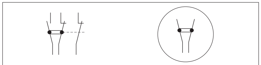
Bild 4: Links: Beispiel für die normgerechte Darstellung von zwangsgeführten Schließer- und Öffnerkontakten und einem nicht zwangsgeführten Öffnerkontakt in einem Schaltplan. Rechts: Beispiel für eine mögliche Kennzeichnung auf dem Gerät, für Geräte, die auch zwangsgeführte Kontakte enthalten.
