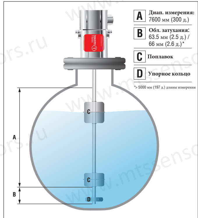
Рис. 4: Монтаж цистерны
