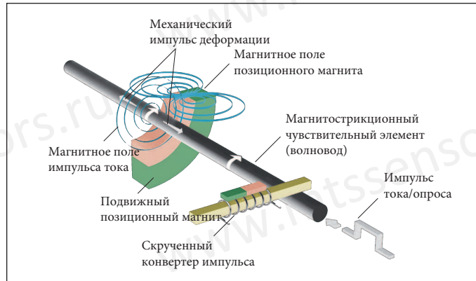
Рис. 1: Магнестрикционный принцип
