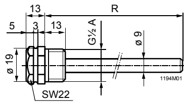
ALT-SB..., ALT-SS...
