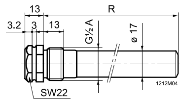
ALT-DS...J
