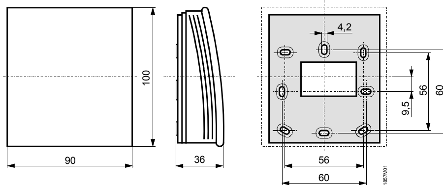
Схема сверления
