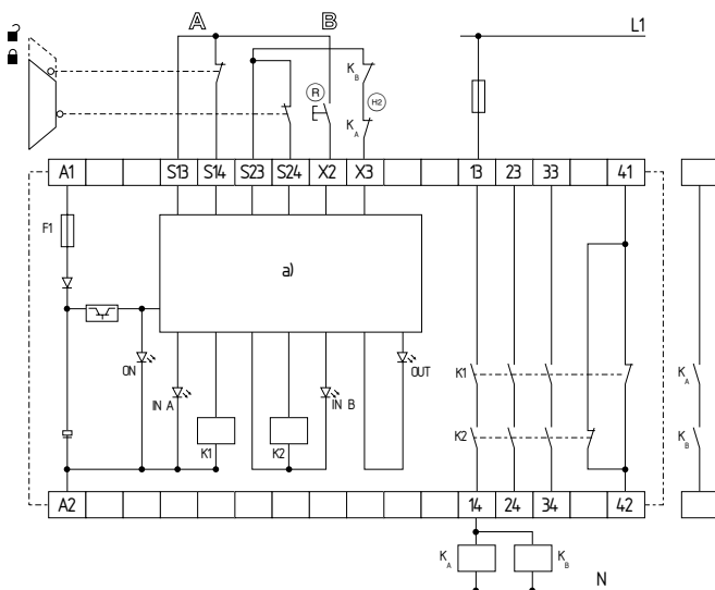
Fig. 2 a) Logic
