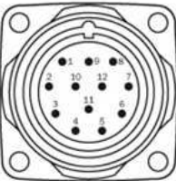
Ansicht Gerätestecker M23, 12-polig am Encoder, SSI
