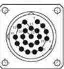
Ansicht Gerätestecker M23, 21-polig am Encoder, Parallel
