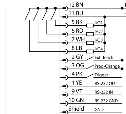
Схема подключения
