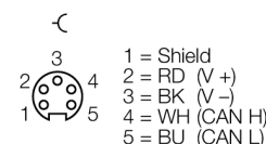
Конфигурация ПИН-контактов справа
