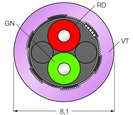
Поперечное сечение проводника
