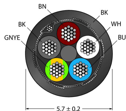
Поперечное сечение проводника
