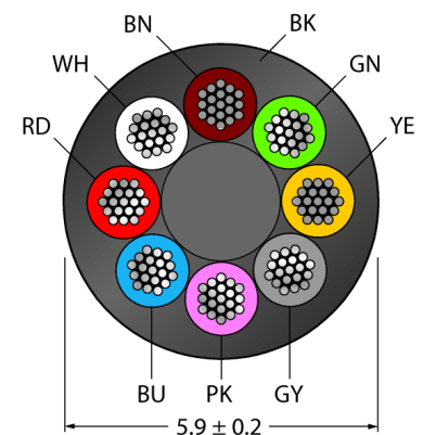
Поперечное сечение проводника
