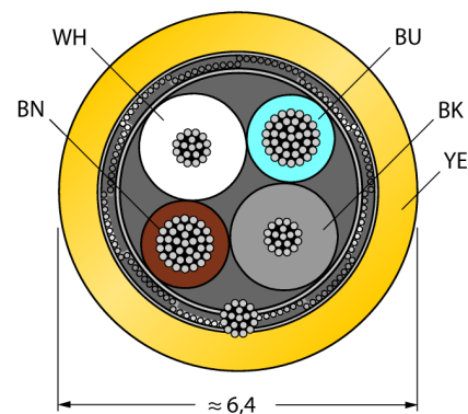
Подпись контактов
