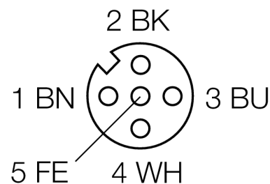
Подпись контактов
