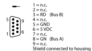
Конфигурация контактов:
