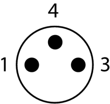
Схема подключения
