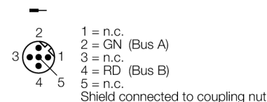
Подпись контактов
